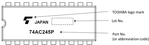
TC74AC245P
