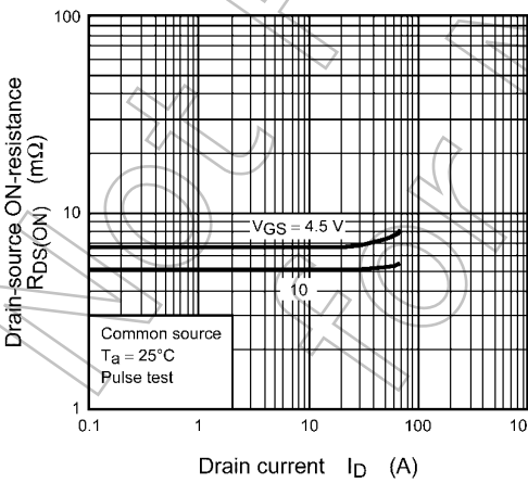
Fig. 8.5 R_{DS(ON)} - I_D
