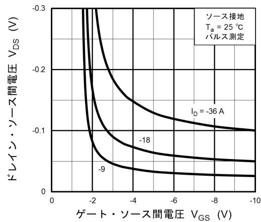
図 8.4 V_{DS} - V_{GS}
