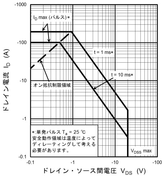
図 8.14 安全動作領域 (最大値 (保証値))
