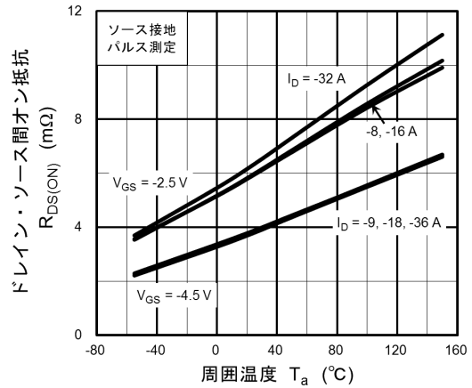
図 8.6 R_{DS(ON)} - T_a
