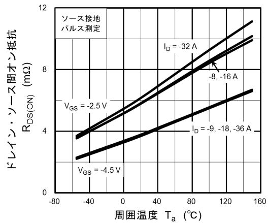
図 8.6 R_{DS(ON)} - T_a
