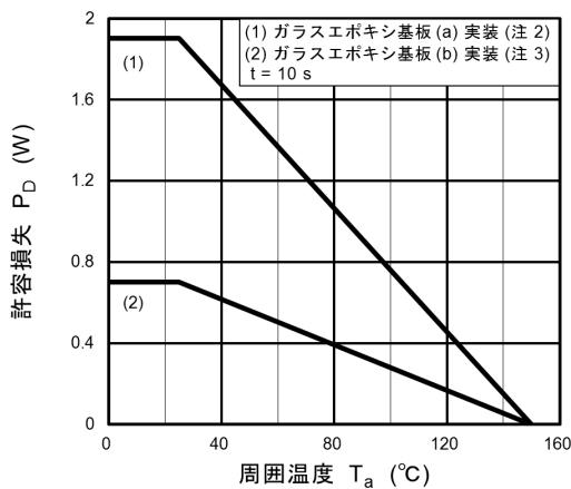
図 8.11 P_D - T_a (最大値 (保証値))
