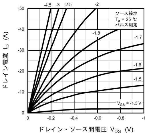
図 8.1 I_D - V_{DS}
