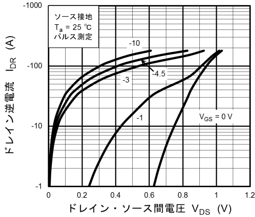
図 8.7 I_{DR} - V_{DS}
