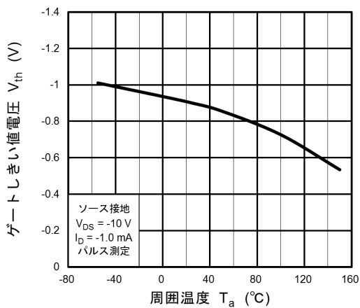
図 8.9 V_{th} - T_a
