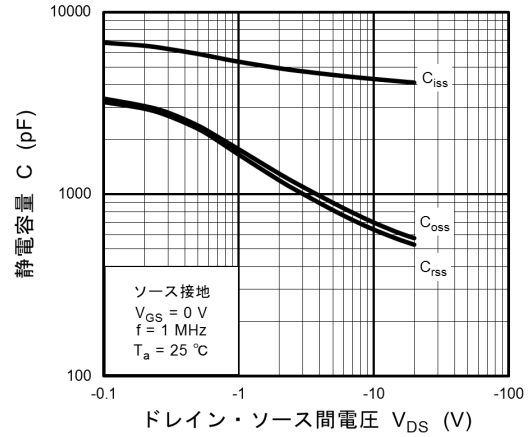
図 8.8 静電容量 - V_{DS}
