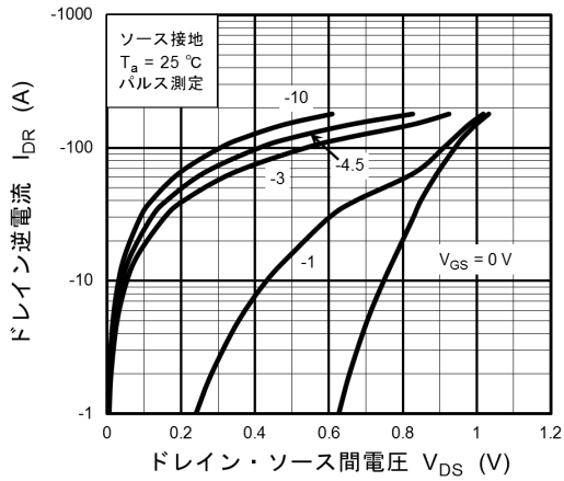
図 8.7 I_{DR} - V_{DS}
