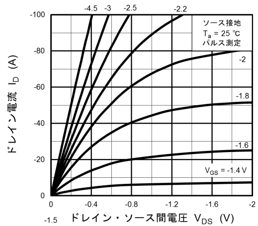
図 8.2 I_D - V_{DS}
