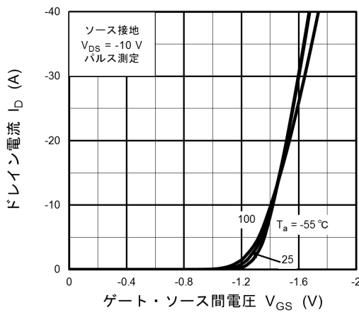
図 8.3 I_D - V_{GS}
