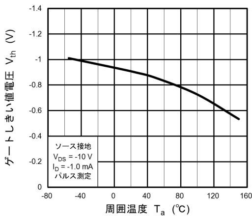
図 8.9 V_{th} - T_a
