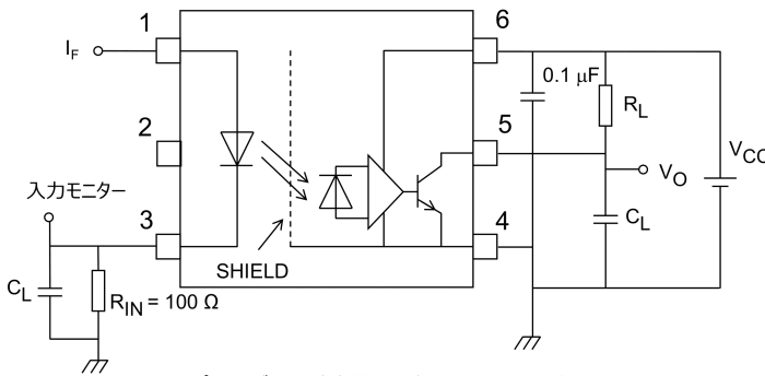
図 13.1.5 伝搬遅延時間測定回路, 波形
