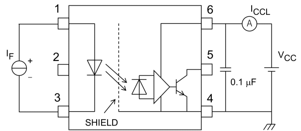
図 13.1.4 I CCL 測定回路
