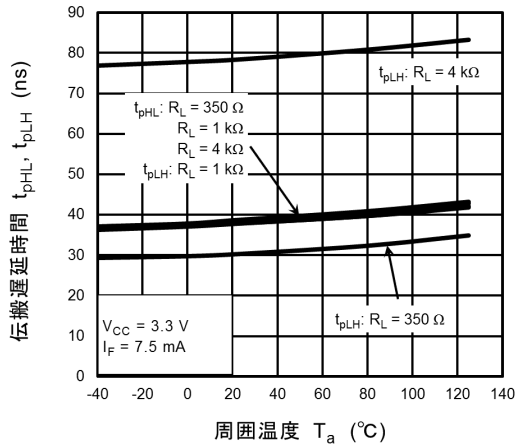
図 13.2.13 t_{pHL}, t_{pLH} - T_a
