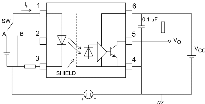
図 13.1.6 コモンモード過渡耐性測定回路, 波形
