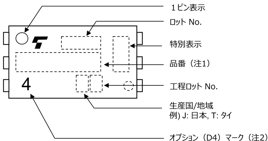
図 17.4 現品表示例
