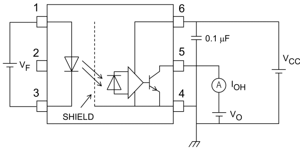
図 13.1.1 I OH 測定回路
