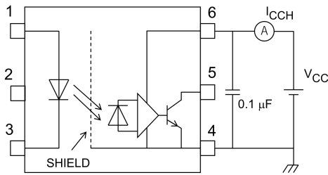
図 13.1.3 I CCH 測定回路
