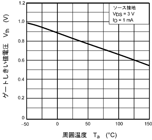
図 7.7 V_{th} - T_a
