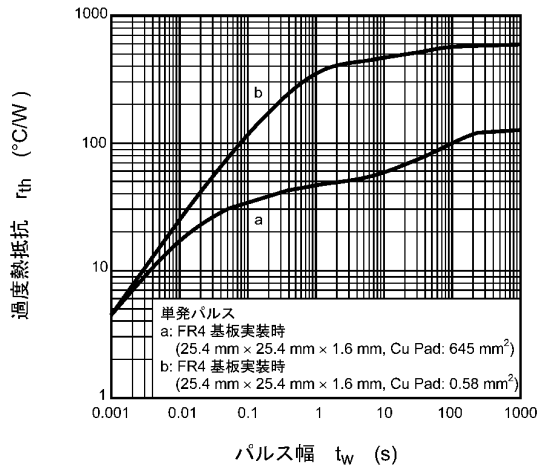
図 7.13 r_{th} - t_w
