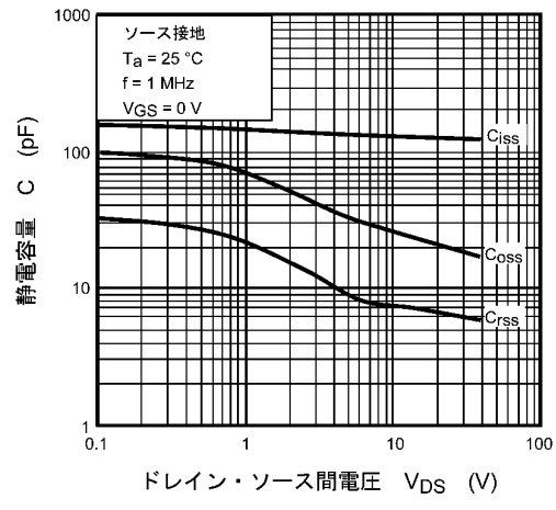
図 7.10 C - V_{DS}
