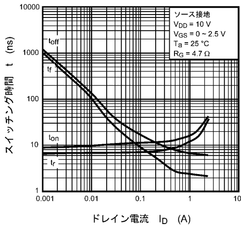
図 7.11 t - I_D
