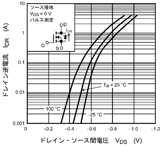
図 7.9 I_{DR} - V_{DS}
