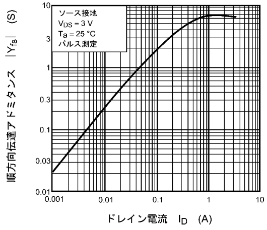
図 7.8 |Y_{fs}| - I_D
