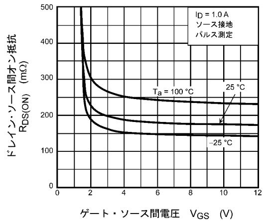
図 7.4 R_{DS(ON)} - V_{GS}
