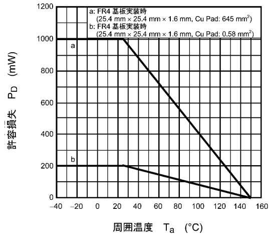
図 7.14 P_D - T_a
