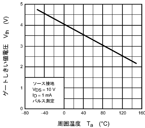
図 8.11 V_{th} - T_a
