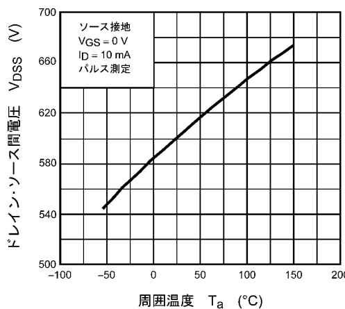
図 8.5 V_{DS} - T_a
