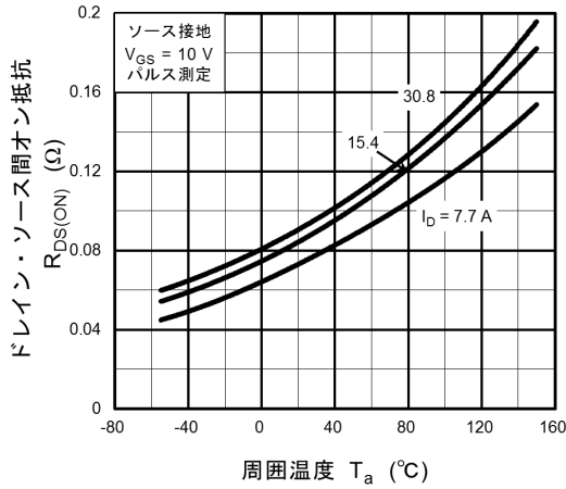
図 8.7 R_{DS(ON)} - T_a
