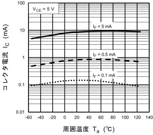
図 11.13 I_C - T_a
