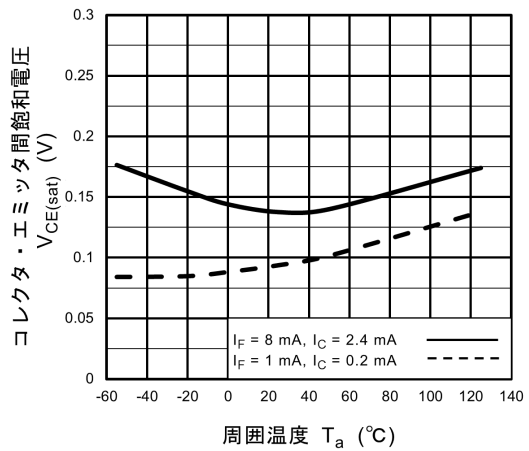
図 11.10 V_{CE(sat)} - T_a
