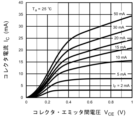
図 11.8 I_C - V_{CE}
