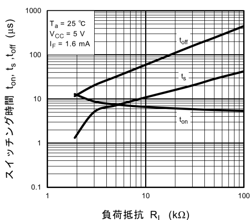
図 11.15 スイッチング時間 - R_L
