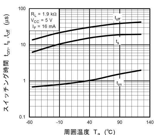
図 11.16 スイッチング時間 - T_a
