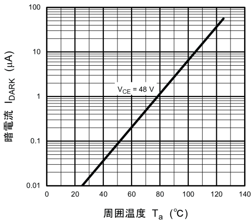
図 11.9 I_{DARK} - T_a
