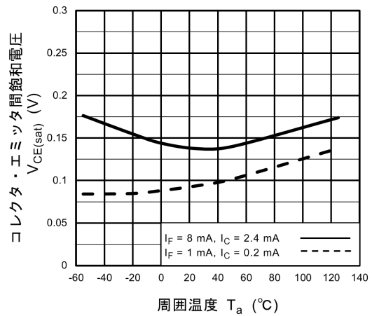
図 11.10 V_{CE(sat)} - T_a
