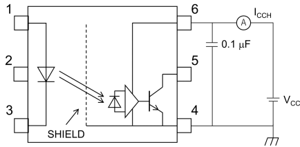
Fig. 13.1.3 I_{CCH} Test Circuit
