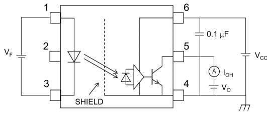
Fig. 13.1.1 I_{OH} Test Circuit
