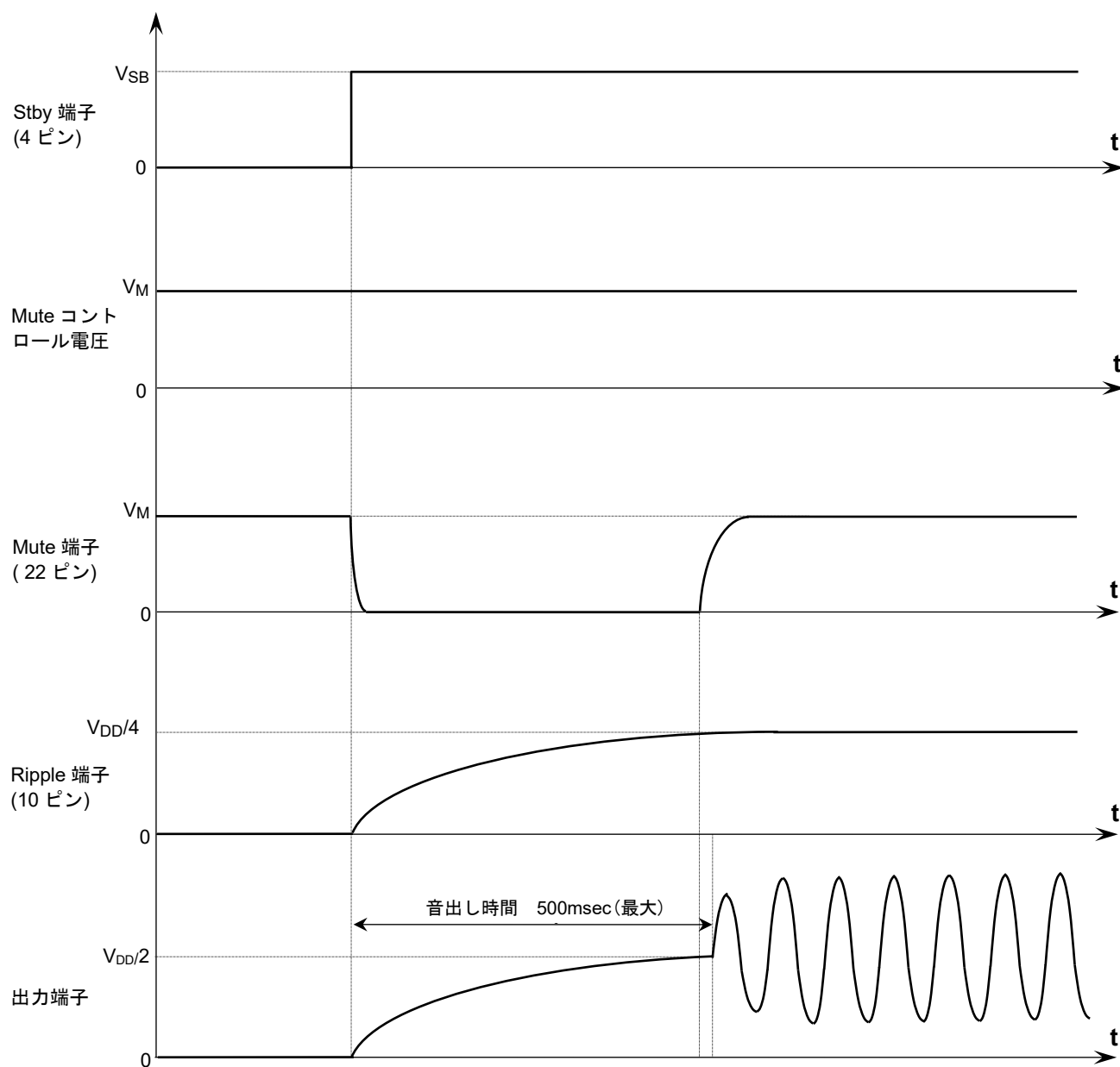
図 5 スタンバイ OFF 時のシーケンス
