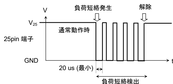
図 10 負荷短絡時 25 ピン出力波形
