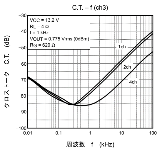
図 17-6 クロストークの周波数特性
