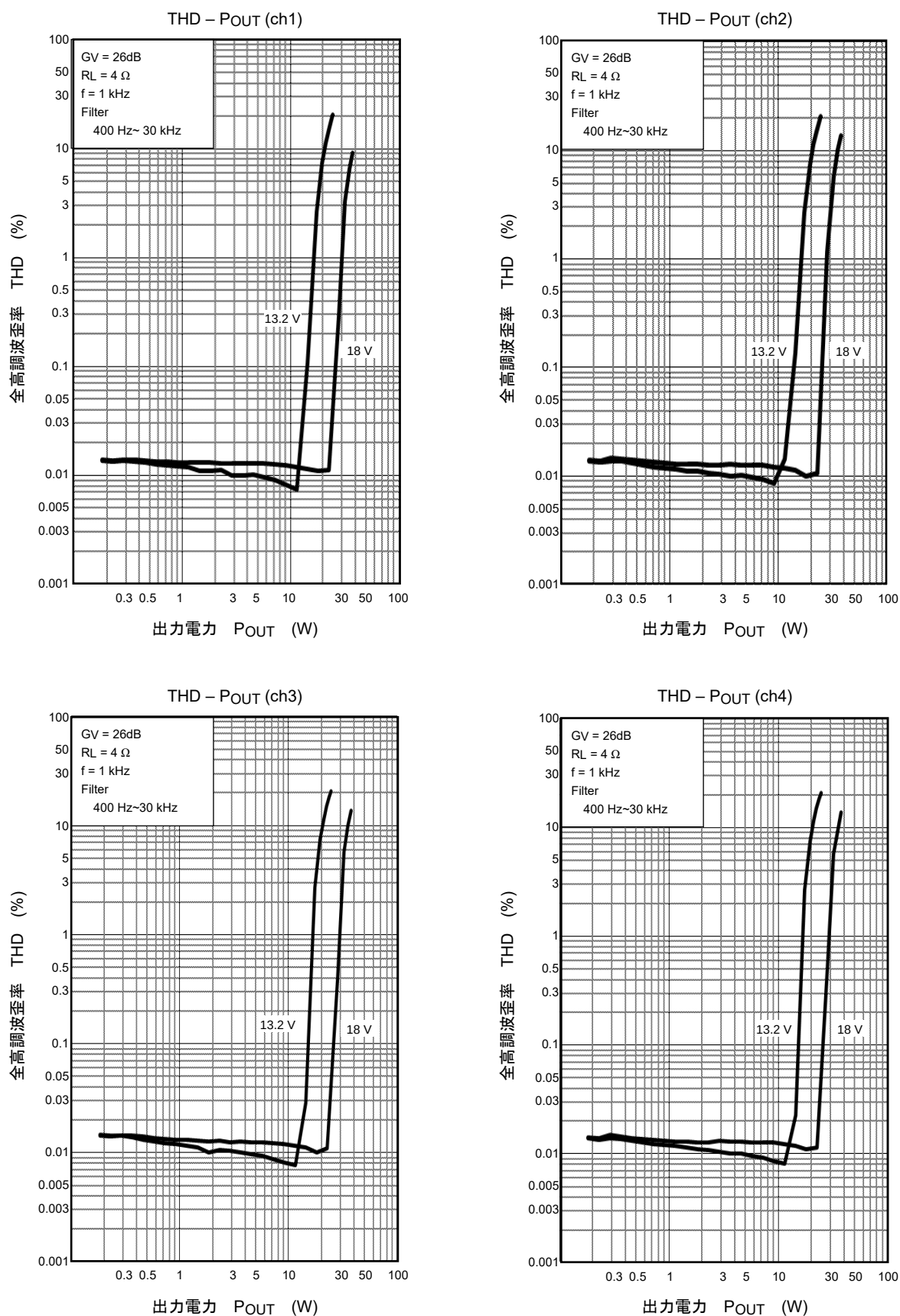
図 17-2 電源電圧による全高調波歪率 ( R_L = 4\ \Omega )
