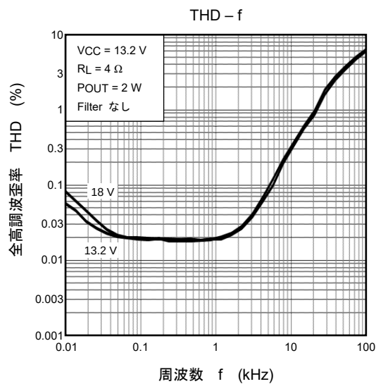
図 17-3 全高調波歪率の周波数特性
