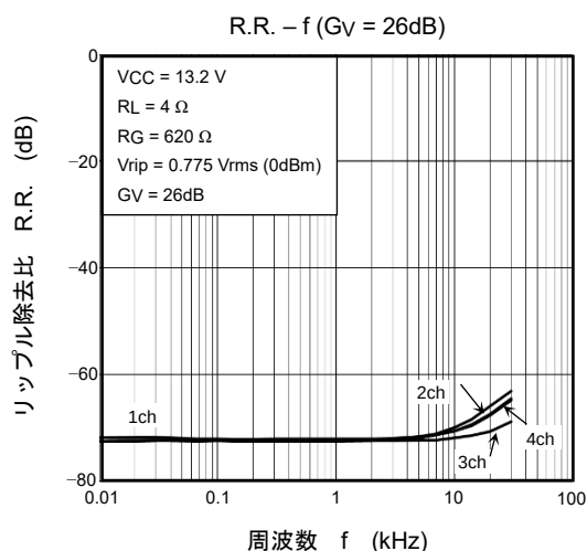
図 17-5 リップル除去比の周波数特性
