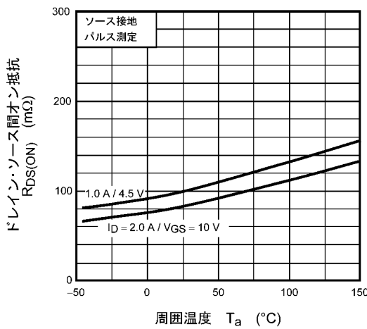
図 8.5 R_{DS(ON)} - T_a
