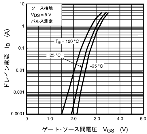
図 8.2 I_D - V_{GS}
