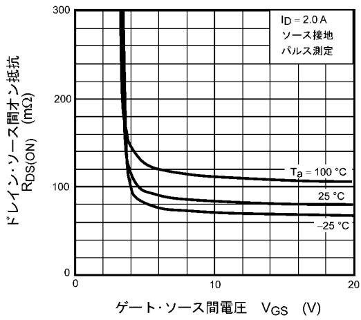
図 8.3 R_{DS(ON)} - V_{GS}
