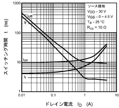
図 8.10 t - I_D
