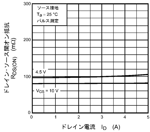
図 7.4 R_{DS(ON)} - I_D
