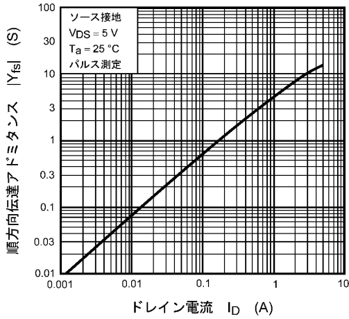
図 8.7 |Y_{fs}| - I_D
