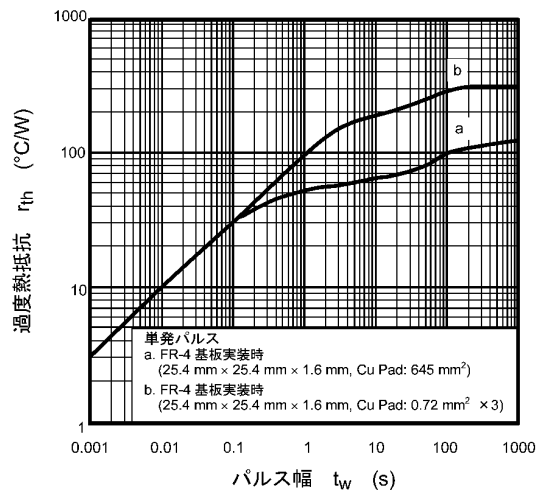
図 7.12 r_{th} - t_w
