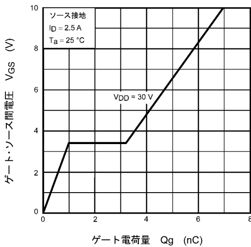
図 8.11 ダイナミック入力特性
