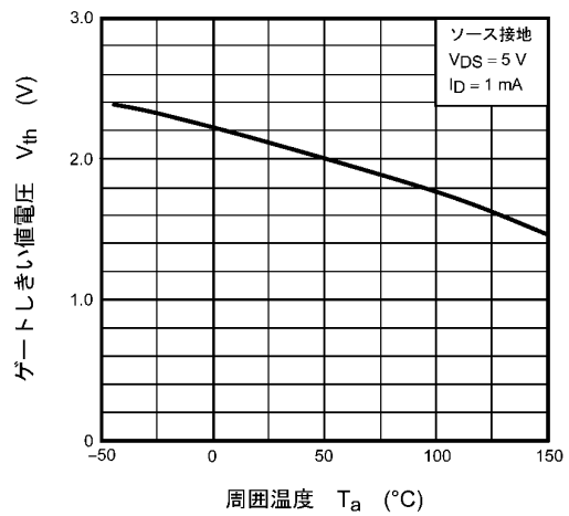
図 7.6 V_{th} - T_a
