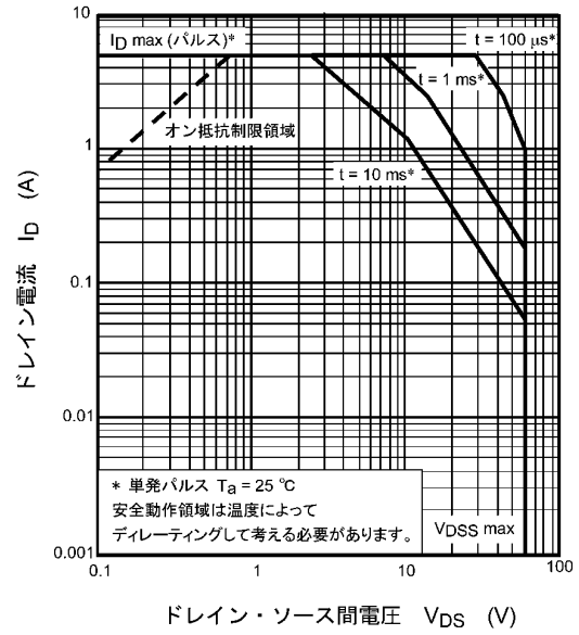
図 8.14 安全動作領域
