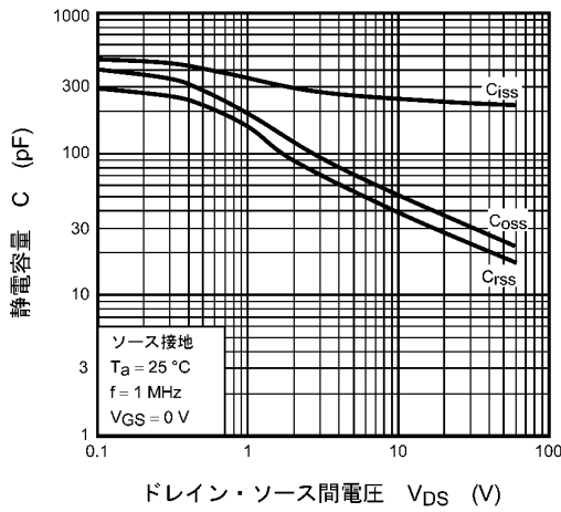
図 7.9 C - V_{DS}
