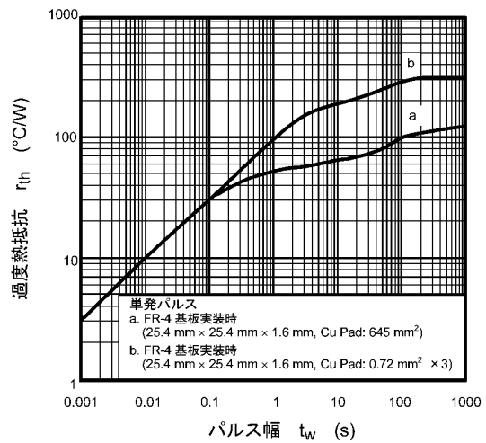
図 8.12 r_{th} - t_w
