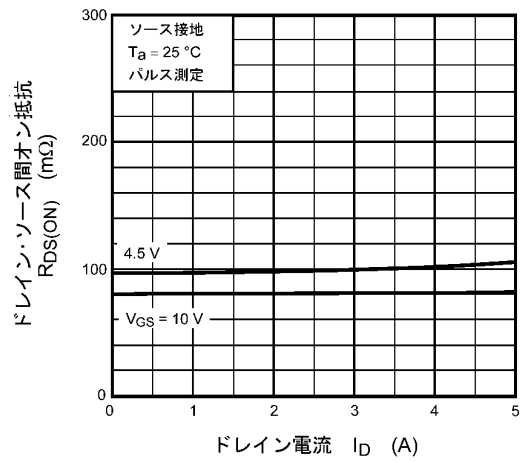
図 8.4 R_{DS(ON)} - I_D
