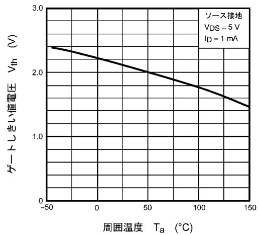
図 8.6 V_{th} - T_a
