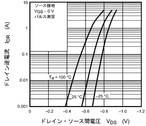
図 8.8 I_{DR} - V_{DS}
