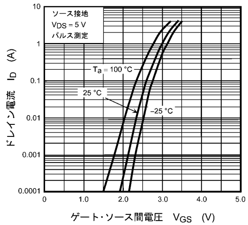
図 7.2 I_D - V_{GS}
