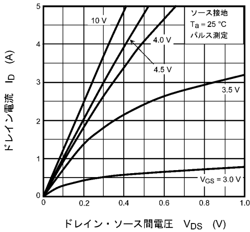
図 7.1 I_D - V_{DS}
