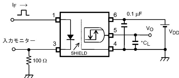
図 12.1.6 伝搬遅延時間測定回路, 波形
