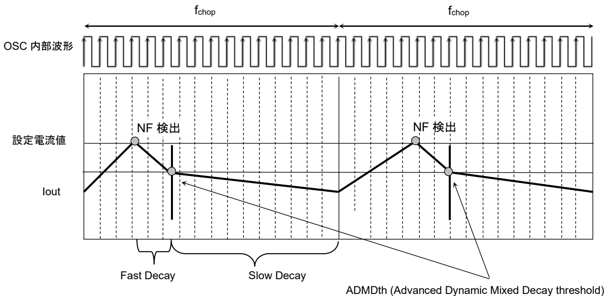
図 6.8 Auto Decay Mode の波形 (電流波形)
