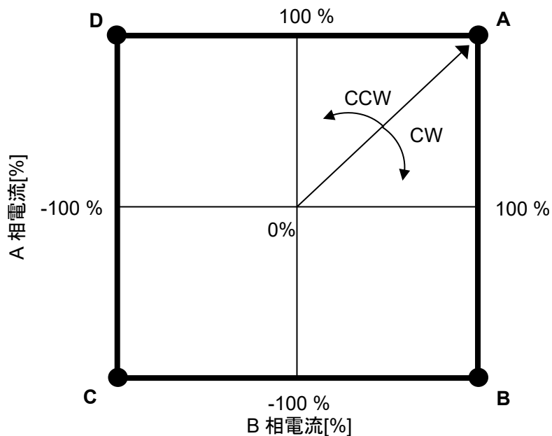
図 6.3 電流ベクトル (1-2 相励磁)
