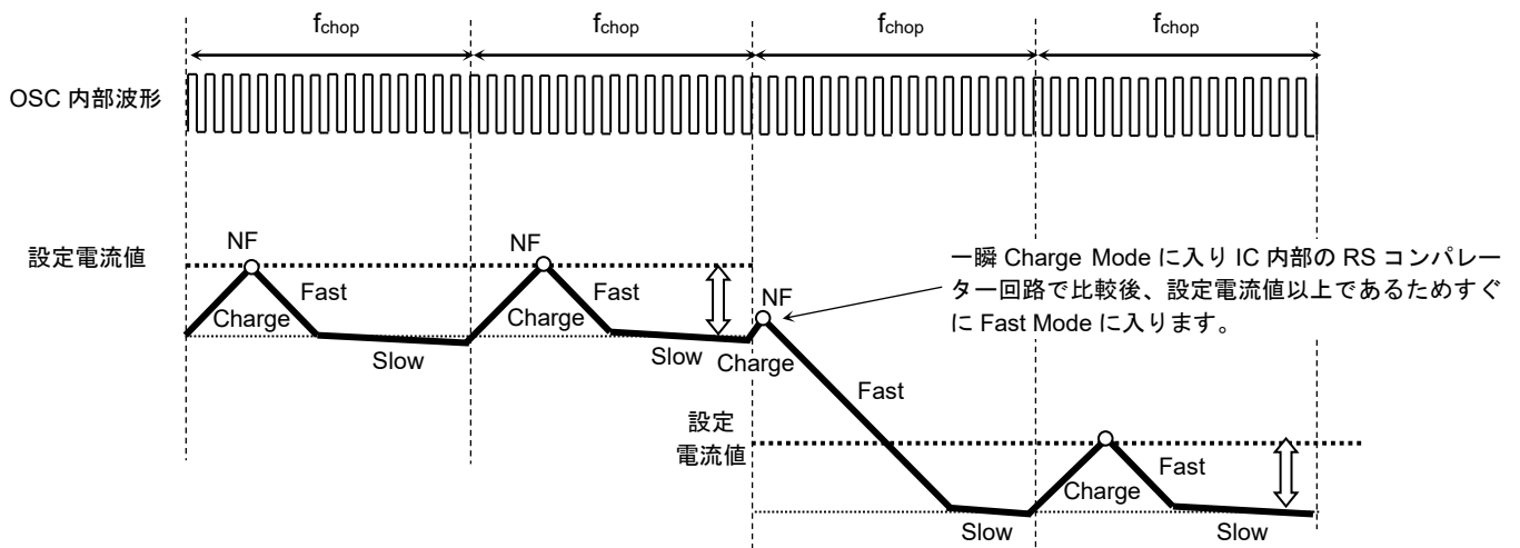
図 6.11 設定電流値が減少方向の場合
