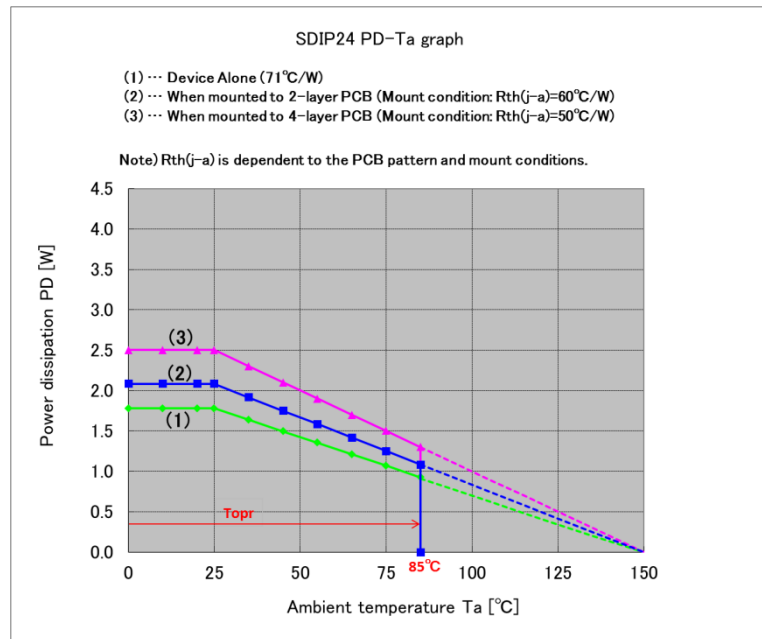
図 7.1 PD-Ta グラフ
