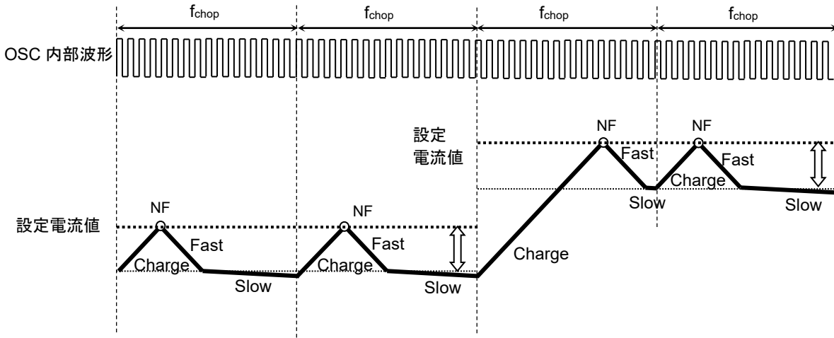
図 6.9 設定電流値が増加方向の場合
