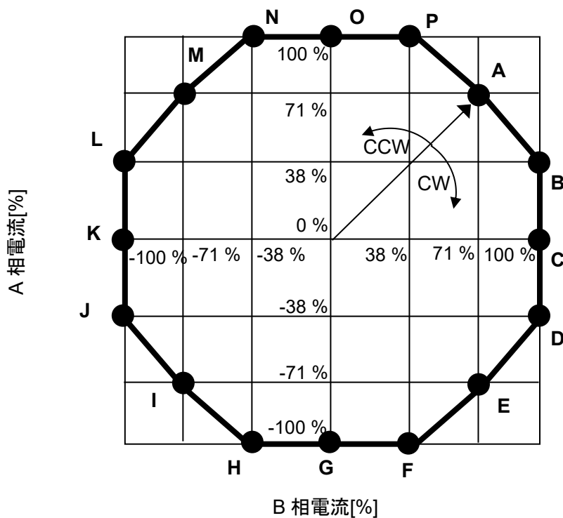
図 6.5 電流ベクトル (W1-2 相励磁)
