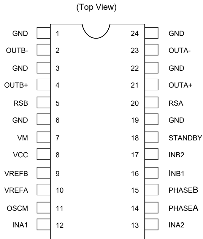
图 4.1 端子配置图
