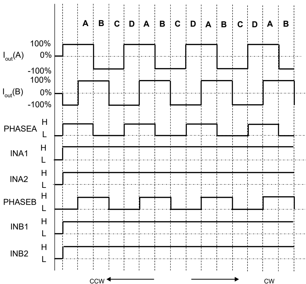
図 6.2 タイミングチャート (2相励磁)
