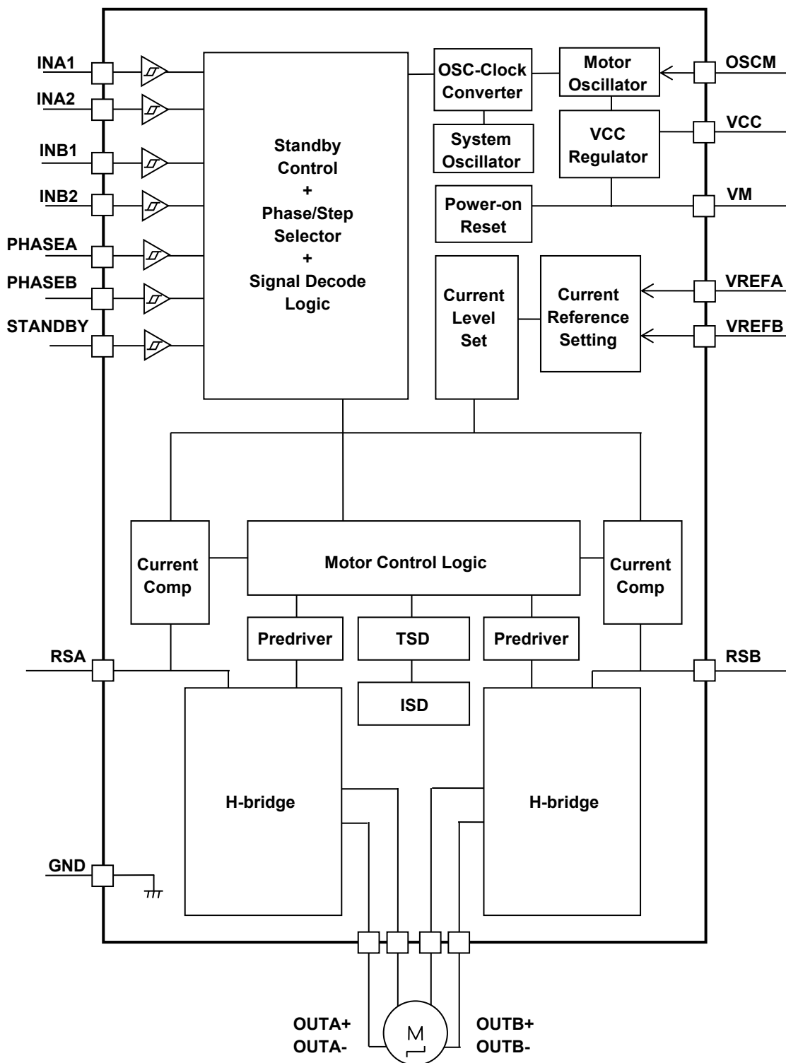
図 3.1 ブロック図
