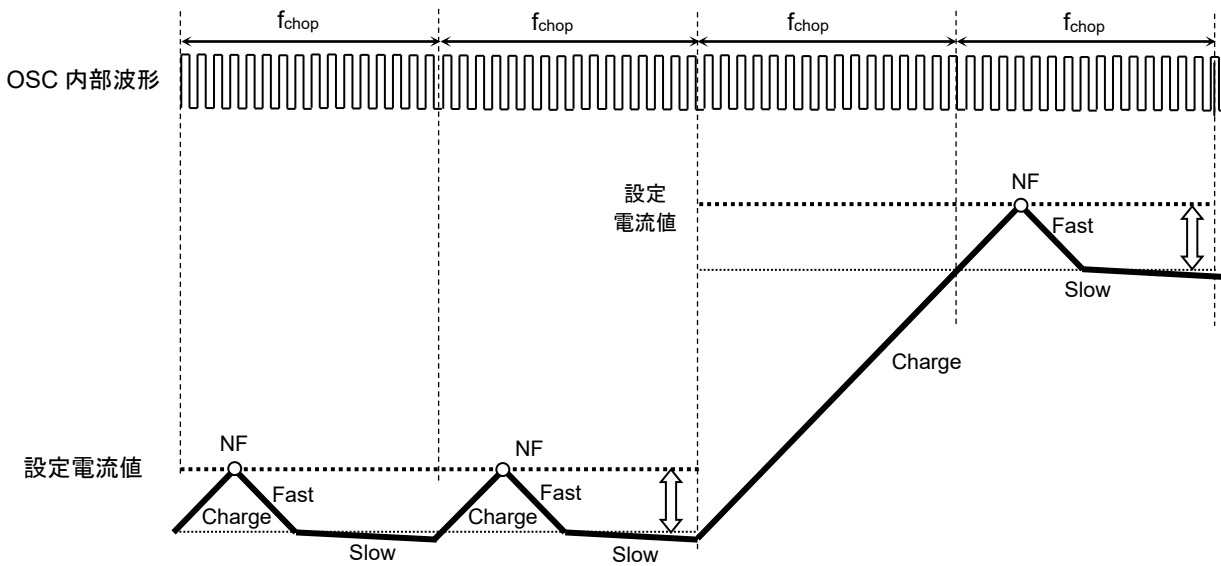
図 6.10 Charge 期間が f_{chop} 1 周期以上の場合
