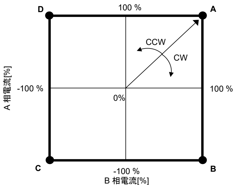
図 6.1 電流ベクトル (2相励磁)
