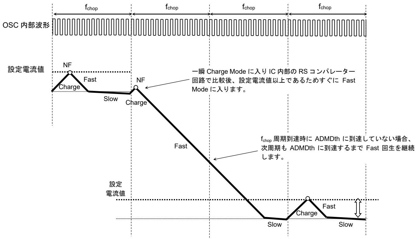
図 6.12 Fast 期間中に f_{chop} 1 周期到達する場合
