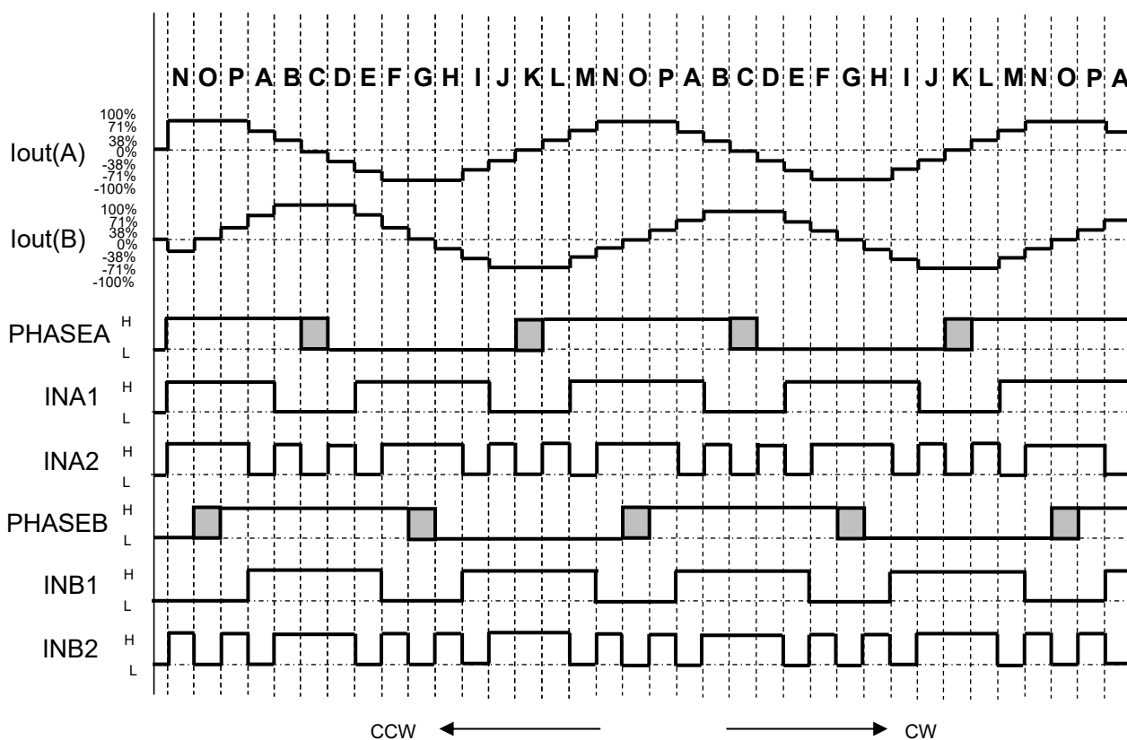
図 6.6 W1-2 相励磁
