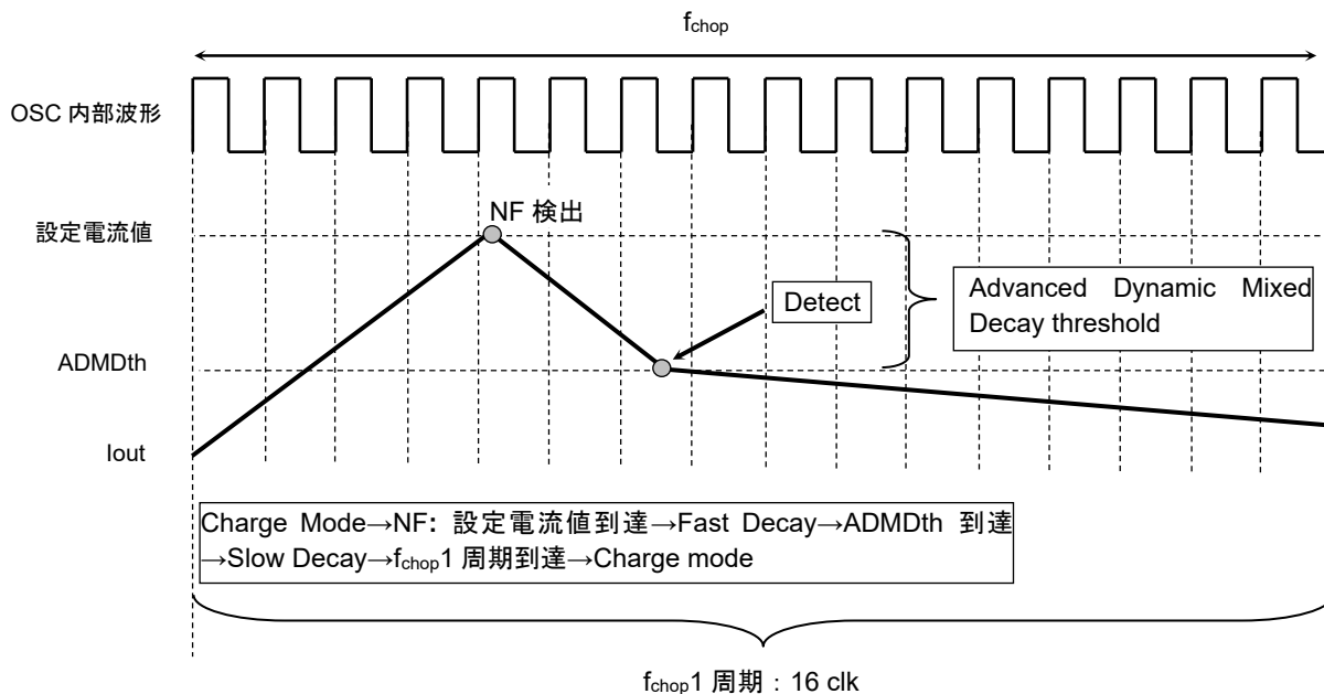
図 6.7 ADMD 定電流制御
