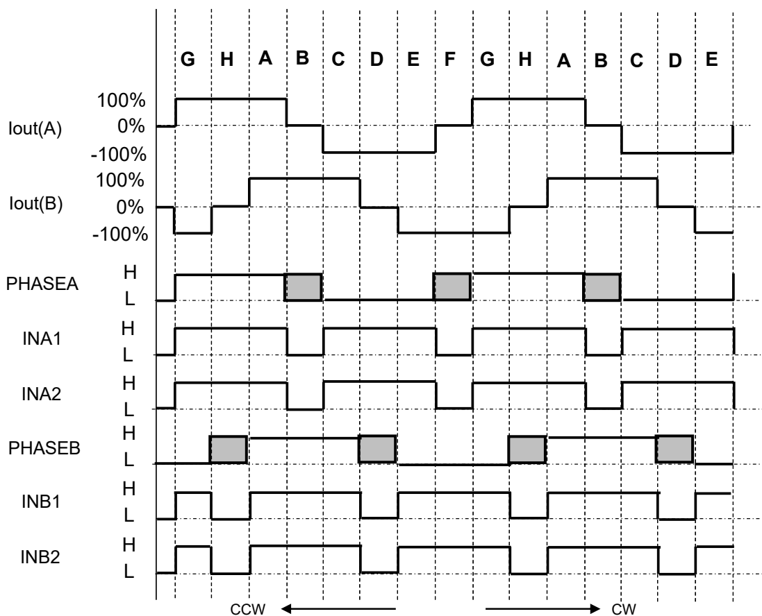
図 6.4 タイミングチャート (1-2 相励磁)
