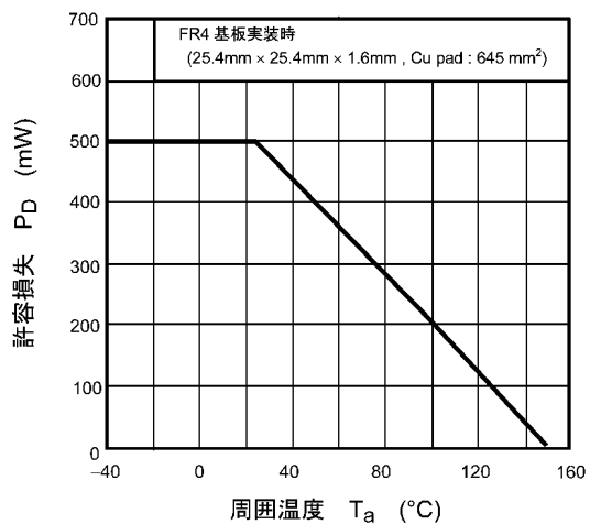
図 7.14 P_D - T_a
