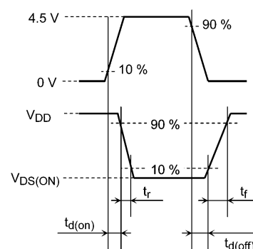
図 5.3.2 入力波形/出力波形
