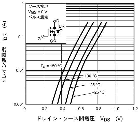
図 7.9 I_{DR} - V_{DS}
