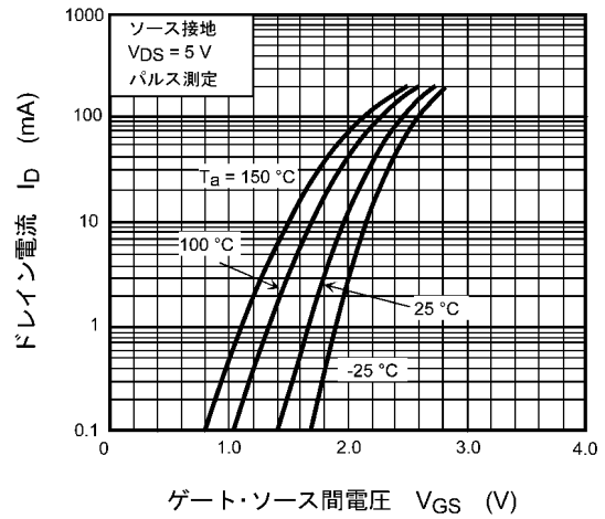
図 7.2 I_D - V_{GS}
