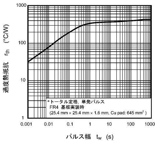
図 7.11 rth - tw
