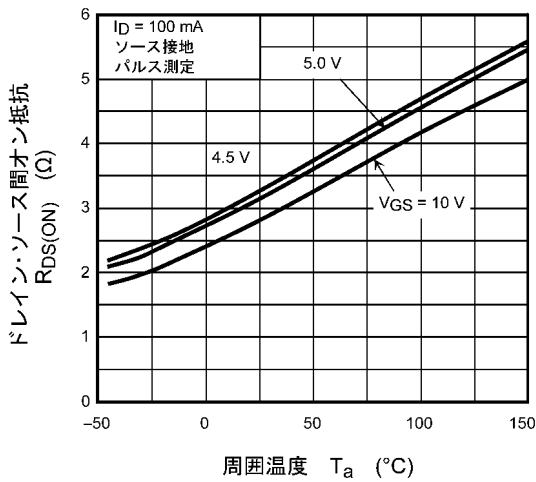
図 7.5 R_{DS(ON)} - T_a
