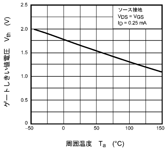
図 7.6 V_{th} - T_a
