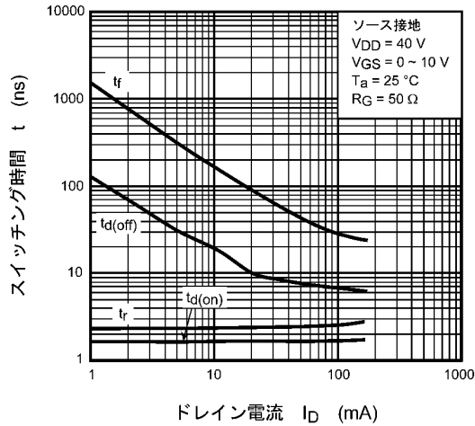
図 7.9 t - ID
