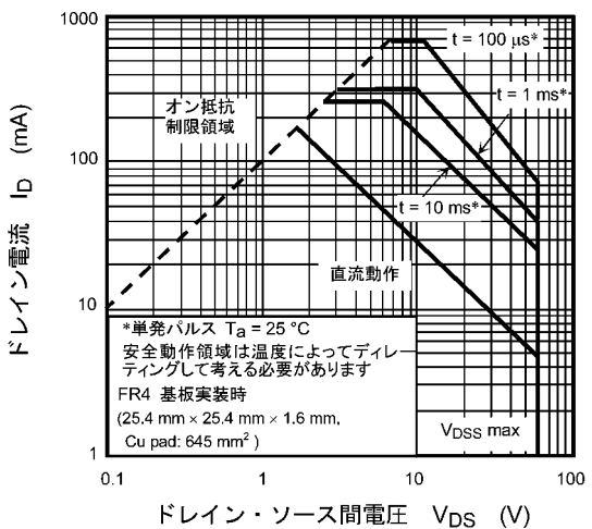
図 7.12 安全動作領域
