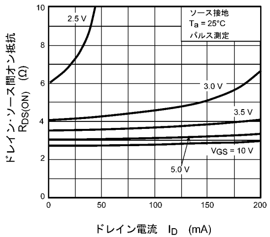
図 7.4 R_{DS(ON)} - I_D
