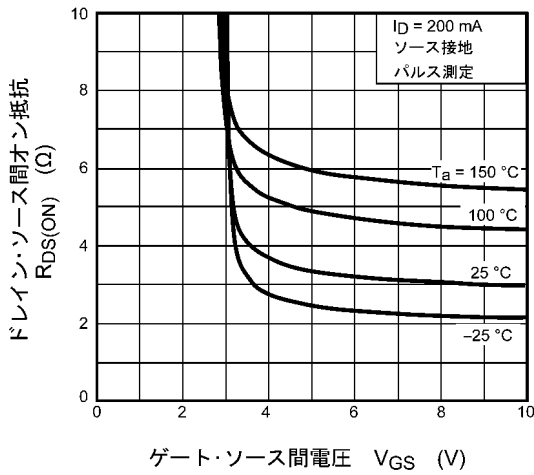
図 7.3 R_{DS(ON)} - V_{GS}
