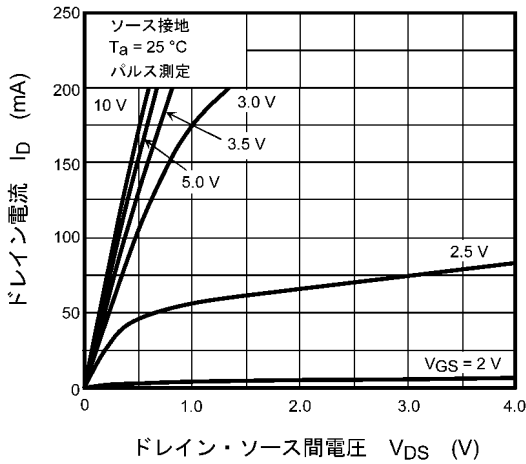
図 7.1 I_D - V_{DS}
