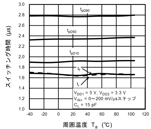
図 12.12 スwitching時間 - T_a
