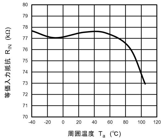
図 12.10 R_{IN} - T_a
