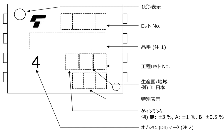
図 16.4 現品表示例
