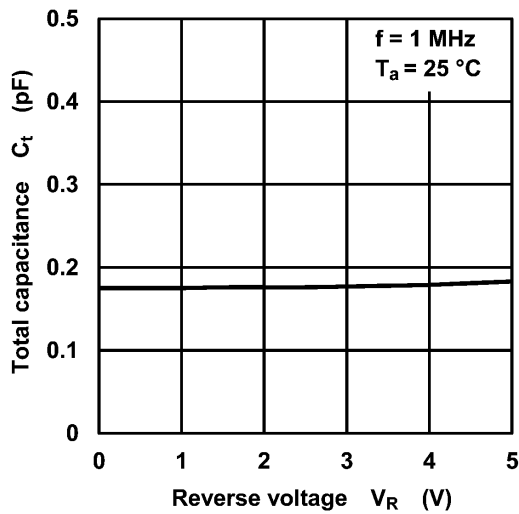
図 7.3 C_t - V_R
