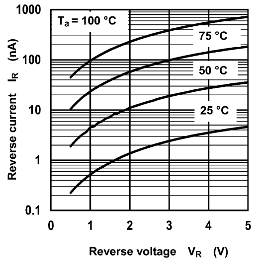
図 7.2 I_R - V_R
