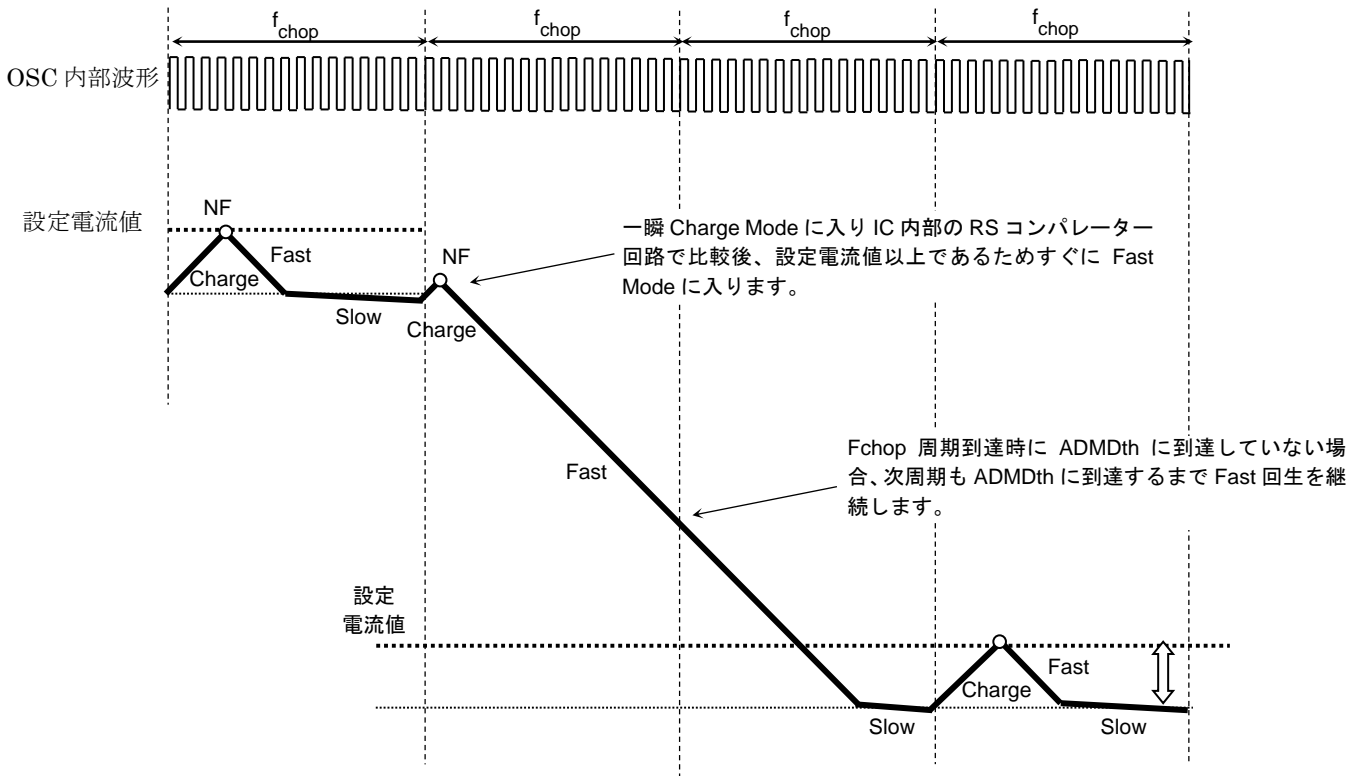
図 6.9 Fast 期間中に fchop 1 周期到達する場合
