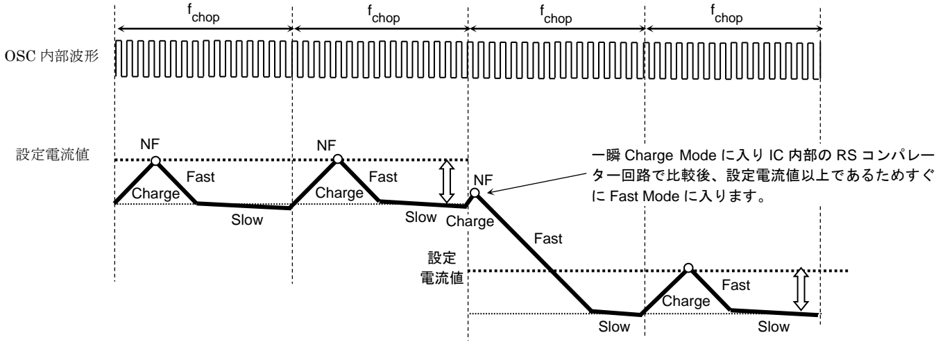
図 6.8 設定電流値が減少方向の場合
