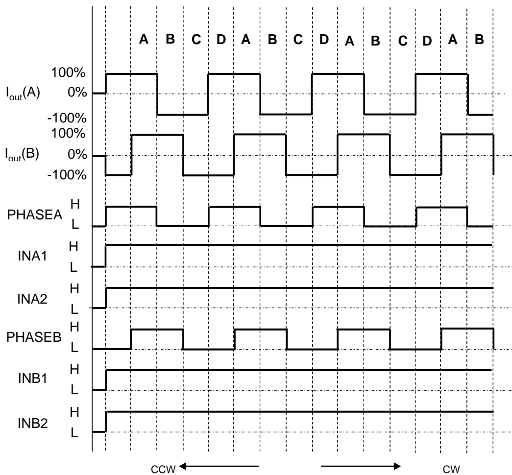
図 6.1 2相励磁
