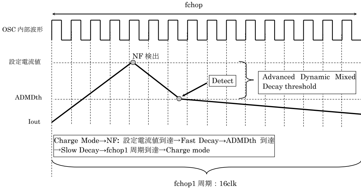
図 6.4 ADMD 定電流制御
