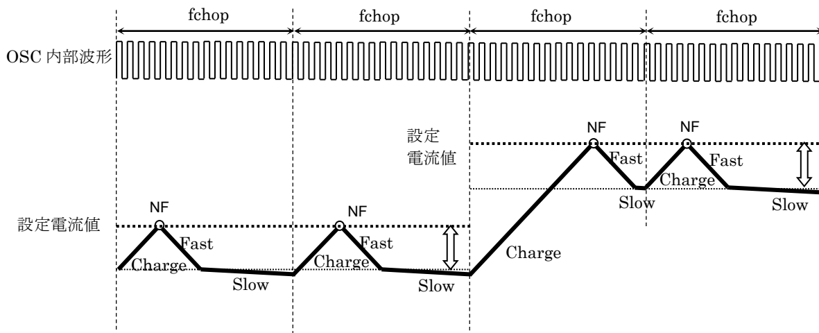
図 6.6 設定電流値が増加方向の場合
