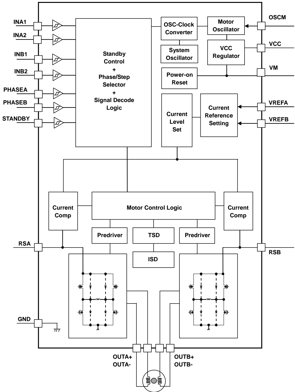
TB67S261 ブロック図
