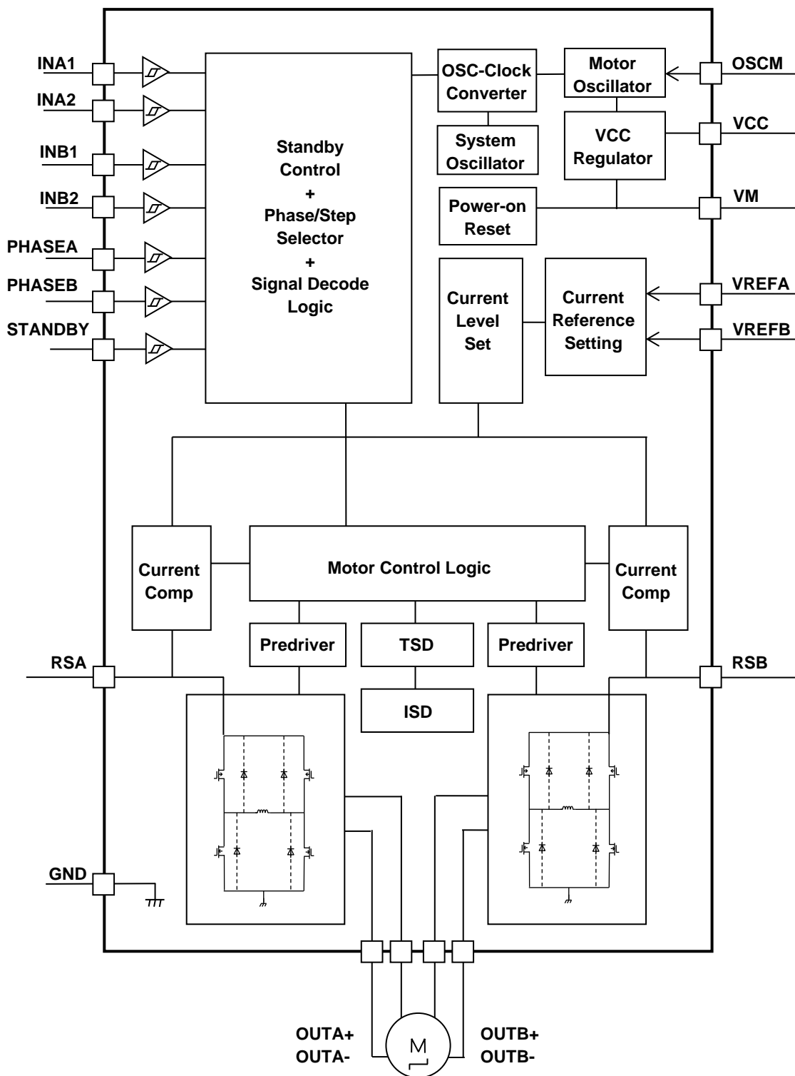
図 3.1 ブロック図
