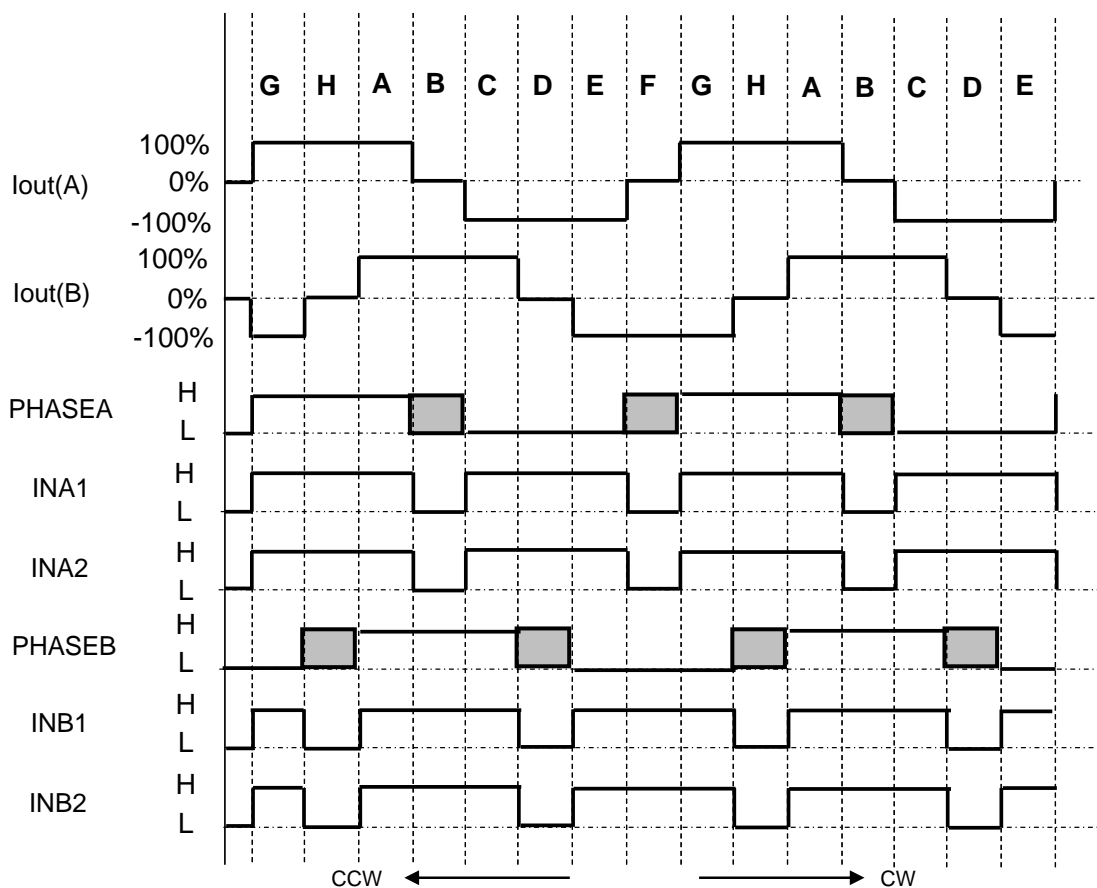
図 6.2 1-2 相励磁
