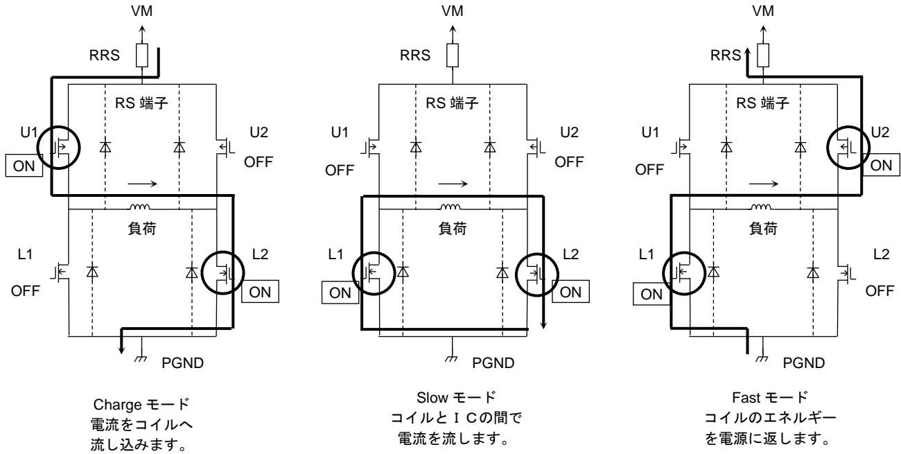
図 6.10 出力段トランジスタ動作モード
