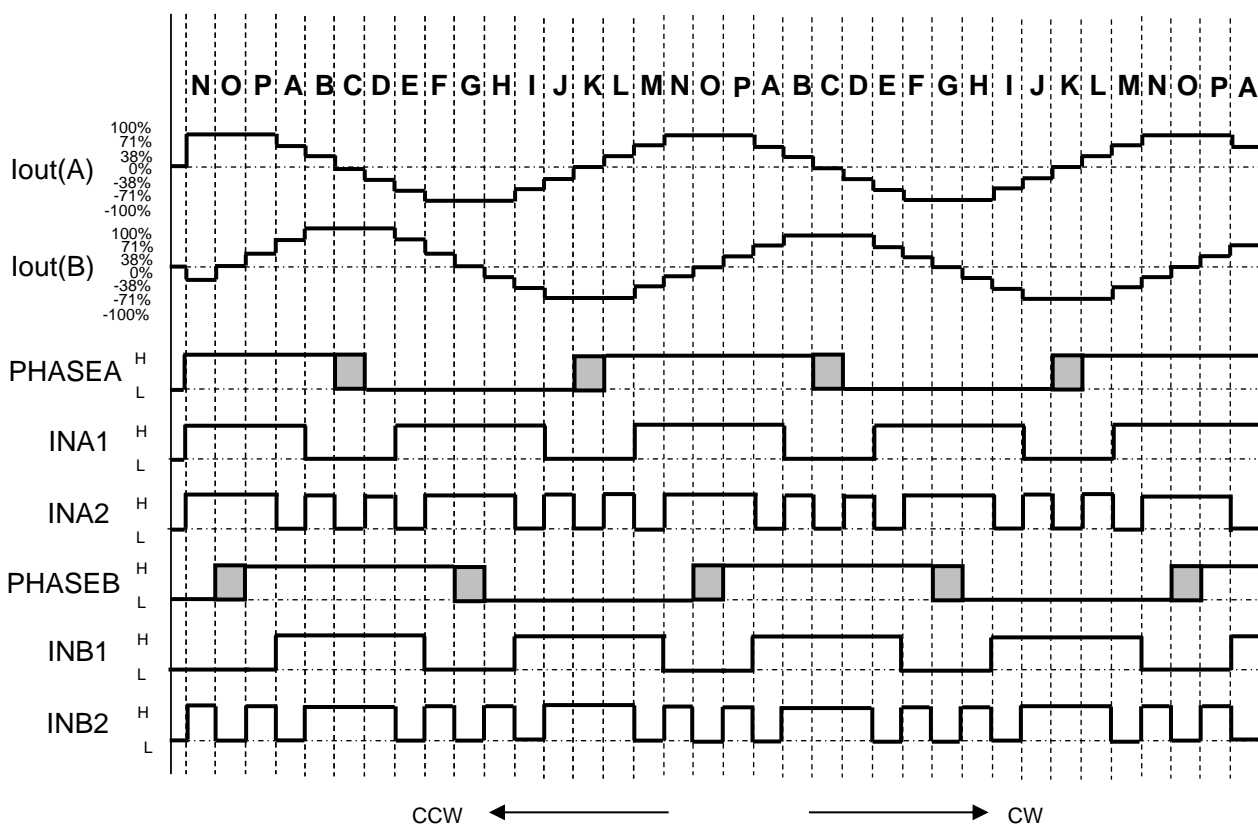
图 6.3 W1-2 相励磁
