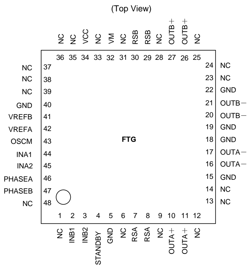
图 4.1 端子配置图
