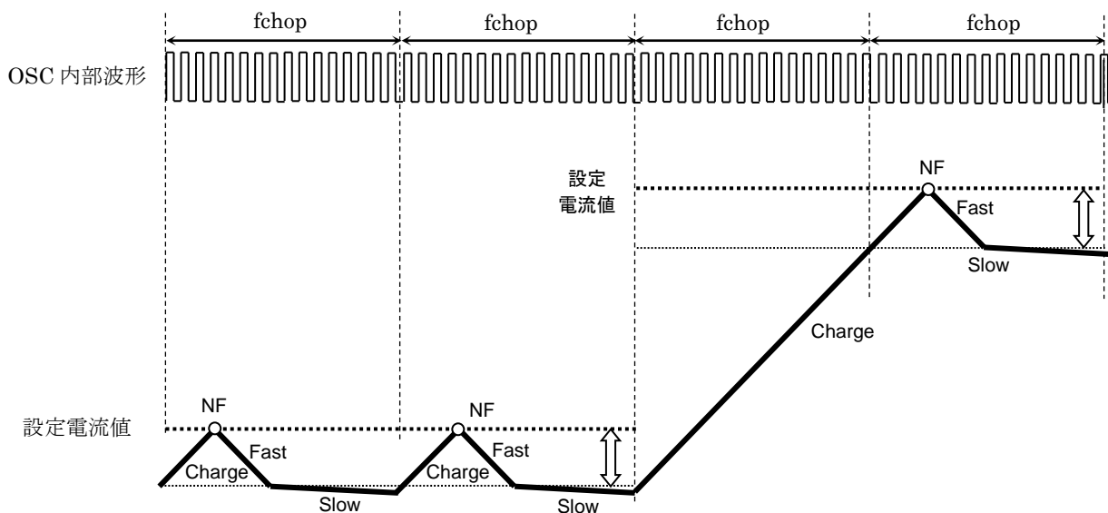
図 6.7 Charge 期間が fchop 1 周期以上の場合
