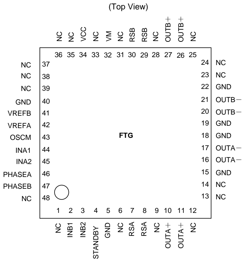
图 4.1 端子配置图
