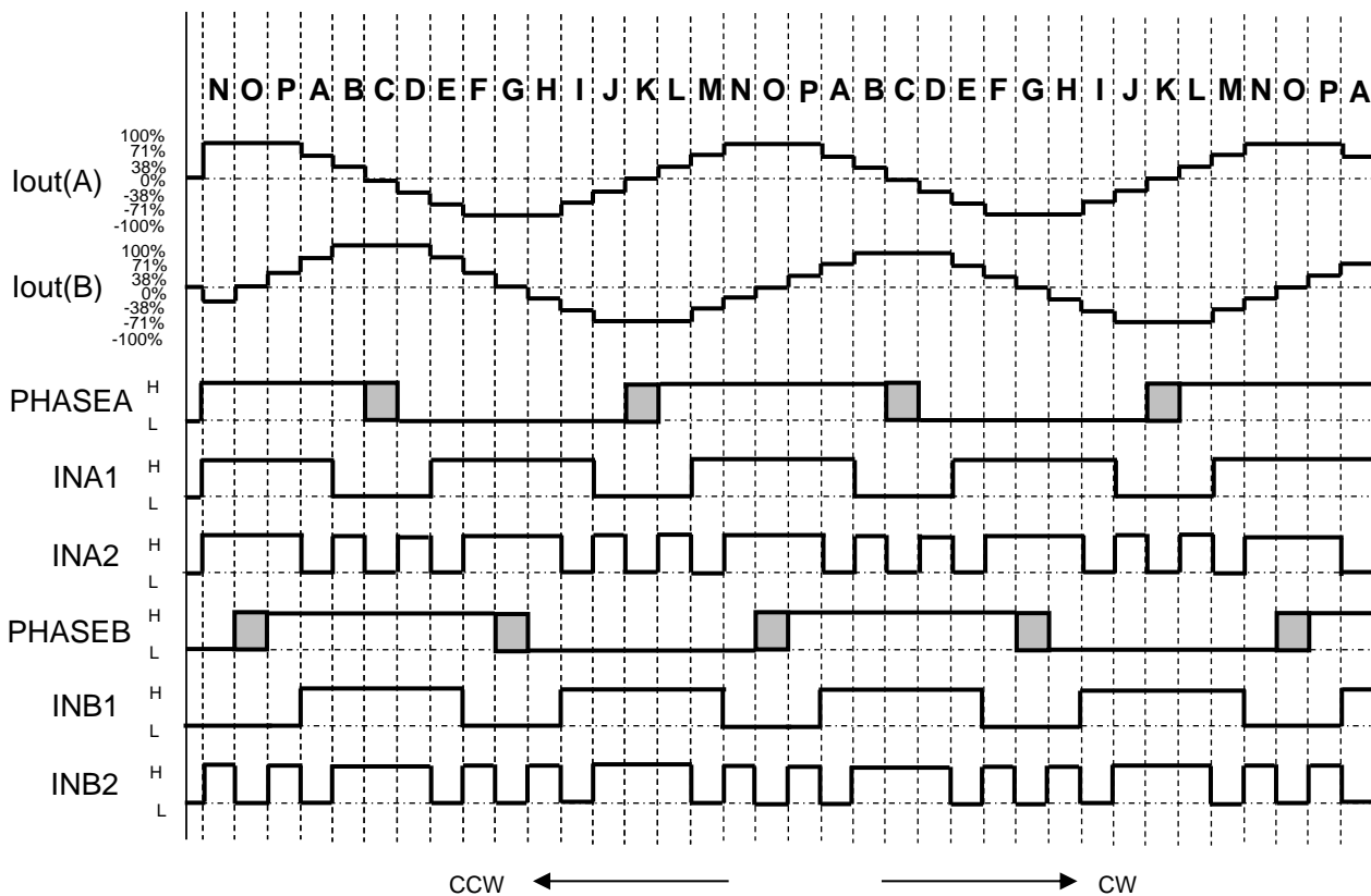
图 6.3 W1-2 相励磁
