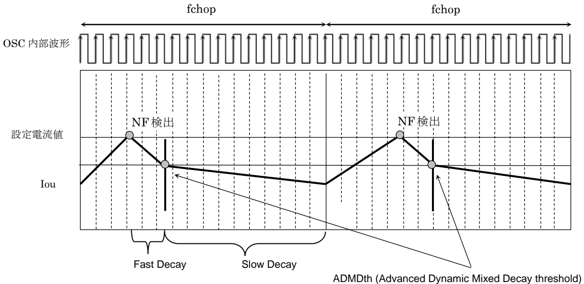
図 6.5 Auto Decay Mode の波形 (電流波形)
