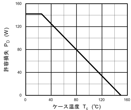
図 8.12 P_D - T_c(\text{Bottom drain}) (最大値 (保証値))
