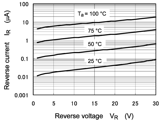
図 9.2 I_R - V_R
