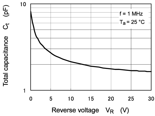
図 9.3 C_t - V_R
