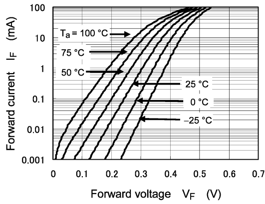
図 9.1 I_F - V_F
