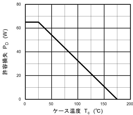
図 8.11 P_D - T_c (最大値 (保証値))
