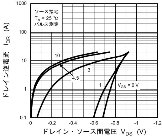
図 8.7 I_{DR} - V_{DS}
