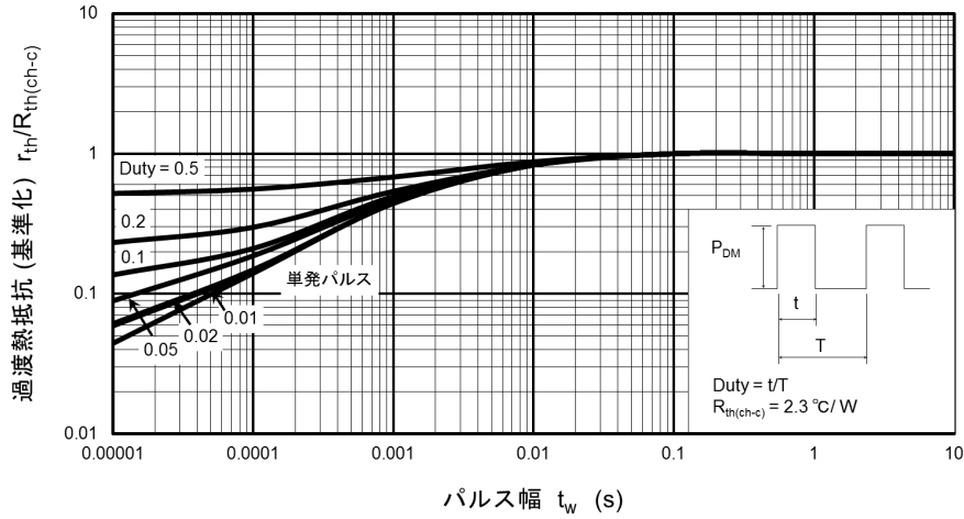
図 8.12 r_{tr}/R_{th(ch-c)} - t_w (最大値 (保証値))
