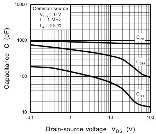
Fig. 8.8 Capacitance - V_{DS}
