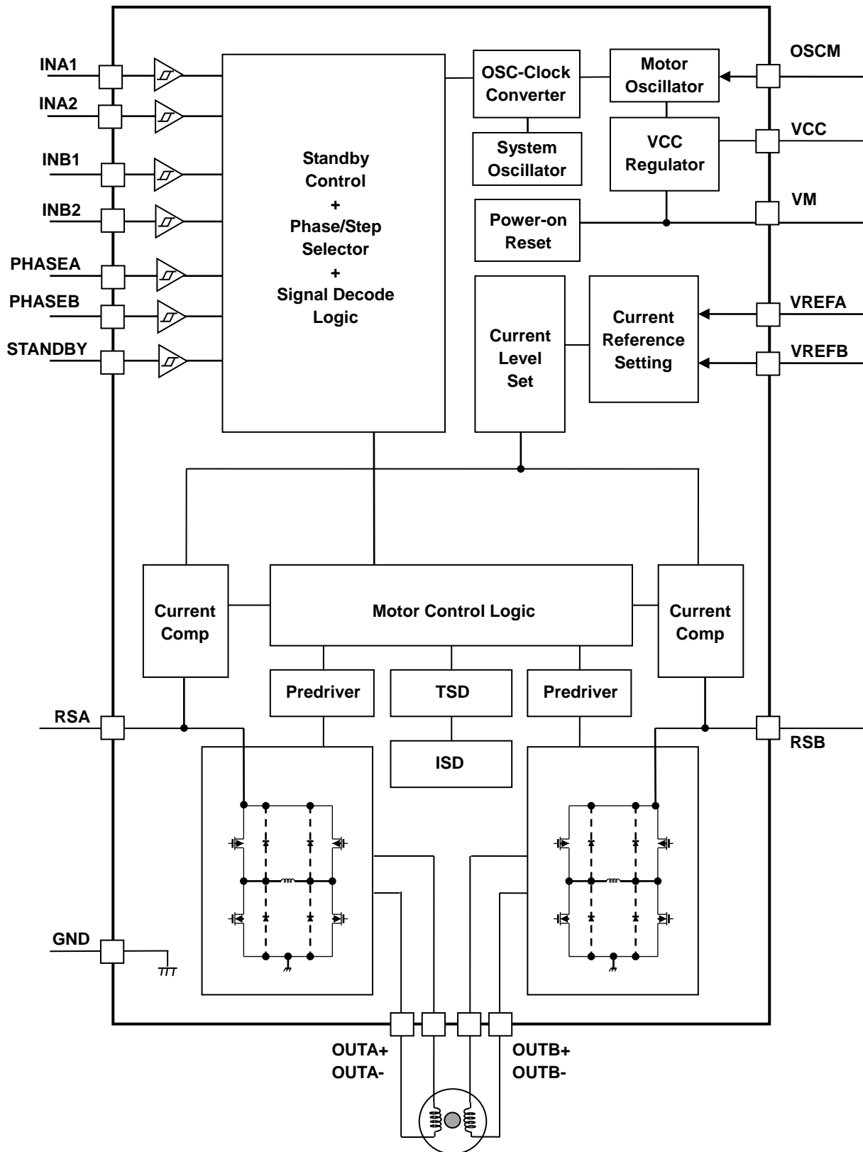
TB62261FTG ブロック図
