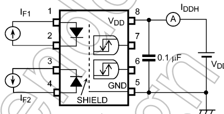
図 12.1.4 IDD_H測定回路
