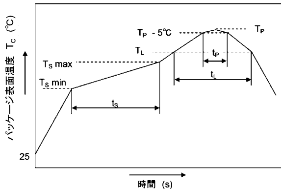
図 13.1.1 鉛フリーはんだ使用時の温度プロファイルー例
