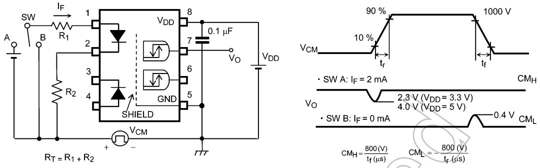
図 12.1.7 コモンモード過渡耐性測定回路, 波形
