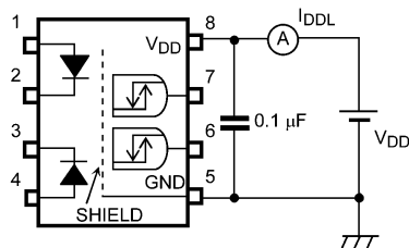
図 12.1.3 IDD_L測定回路
