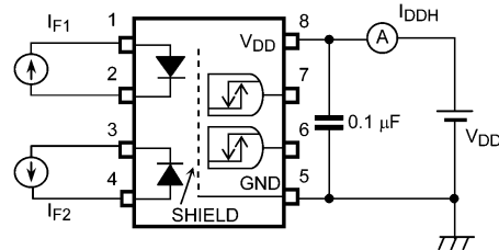
図 12.1.4 IDD_H測定回路
