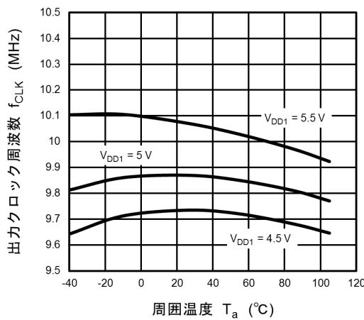
図 12.8 f_{CLK} - T_a
