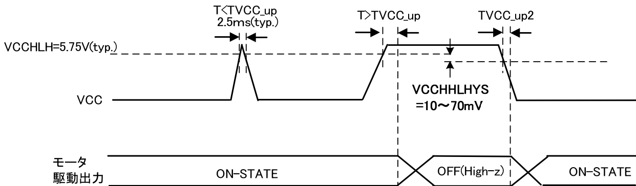
図 7.6.3-2 VCC 高電圧検出タイミングチャート
