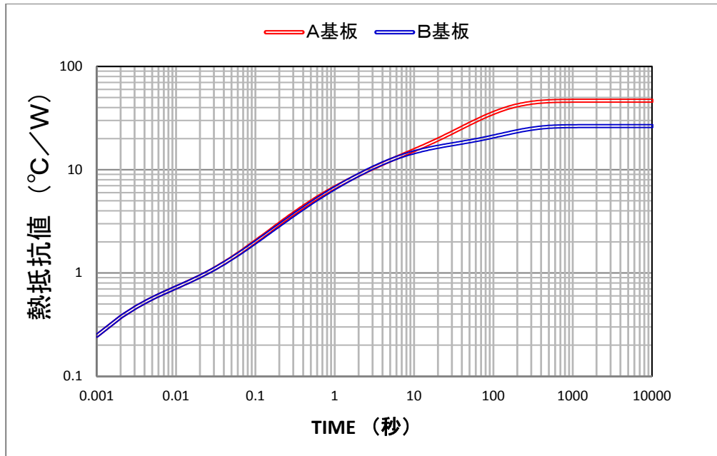
図 8.1 熱抵抗特性
