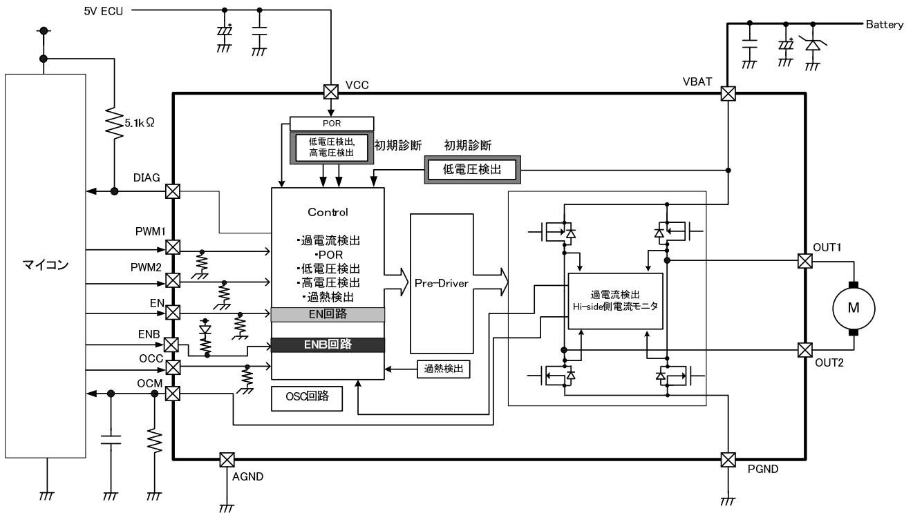
図 4.1 ブロック図
