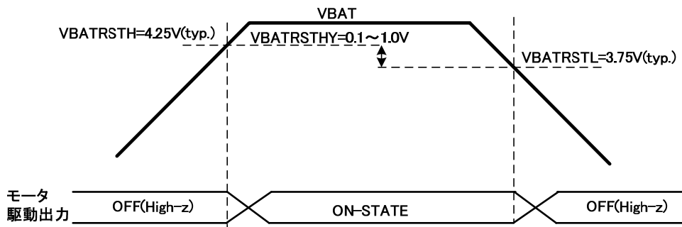
図 7.6.1-1 VBAT 低電圧検出しきい値特性
