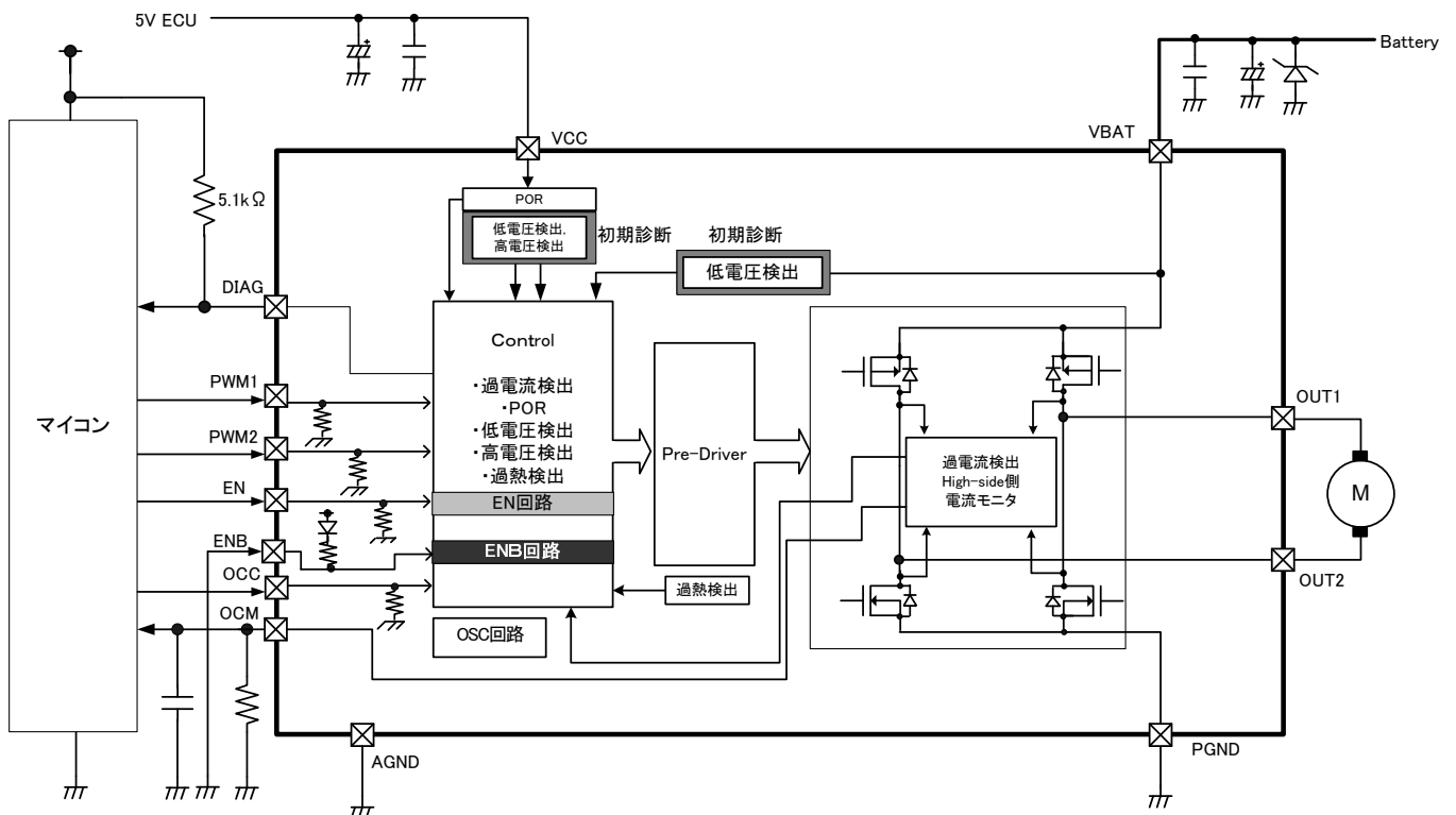
図 12.1 応用回路例 1
