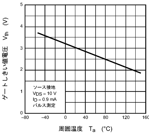
図 8.11 V_{th} - T_a
