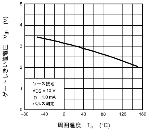
図 8.9 V_{th} - T_a
