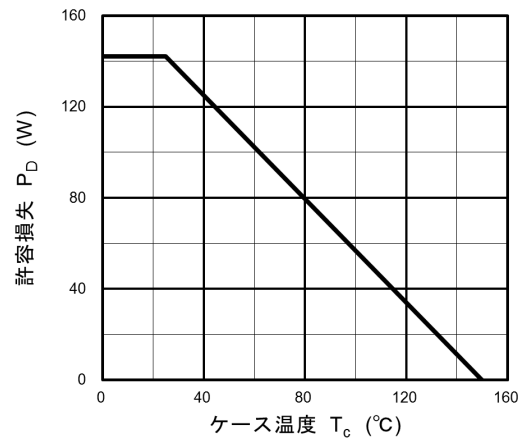
図 8.12 P_D - T_c (Bottom drain) (最大値 (保証値))
