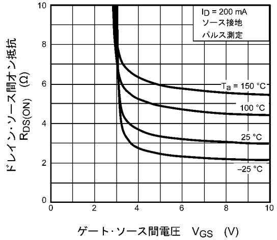
図 8.4 R_{DS(ON)} - V_{GS}
