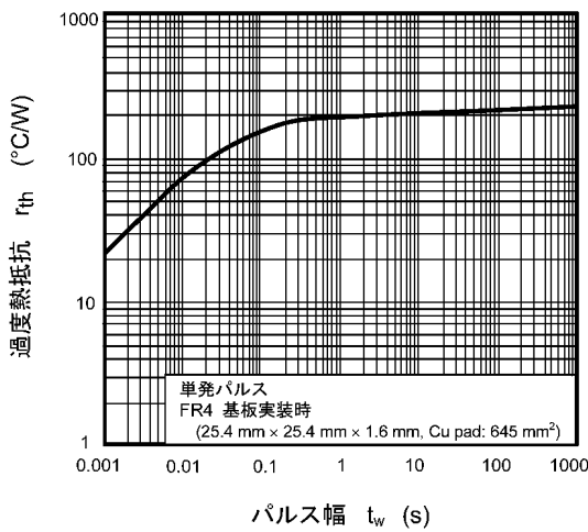
図 8.11 r_{th} - t_w
