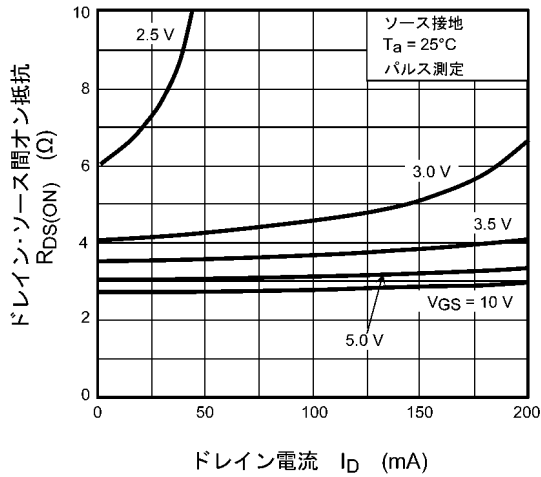
図 8.3 R_{DS(ON)} - I_D
