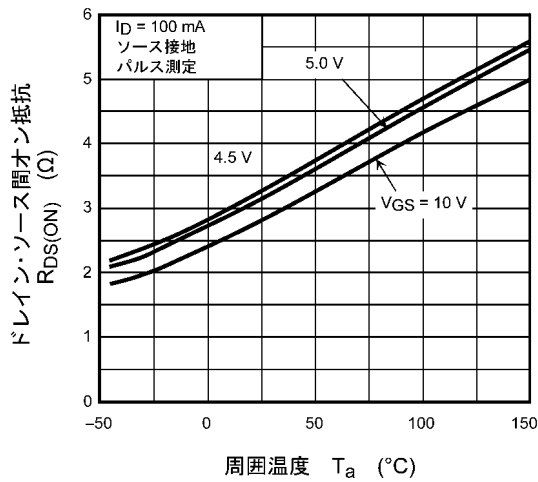
図 8.5 R_{DS(ON)} - T_a
