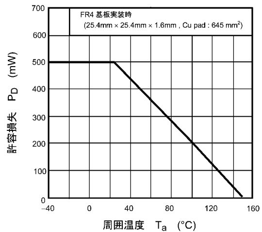
図 8.12 P_D - T_a
