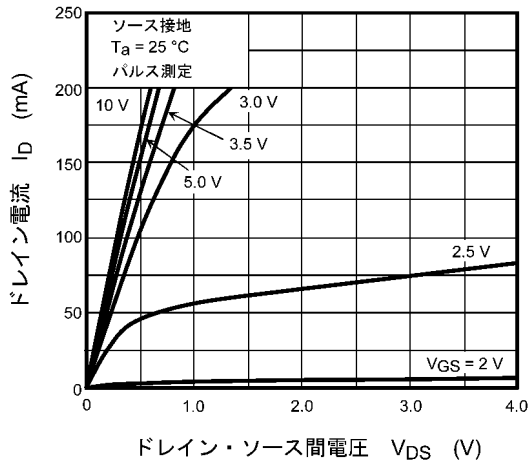
図 8.1 I_D - V_{DS}
