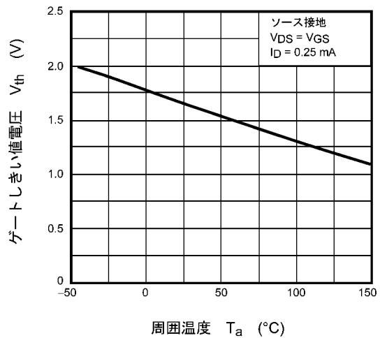
図 8.6 V_{th} - T_a
