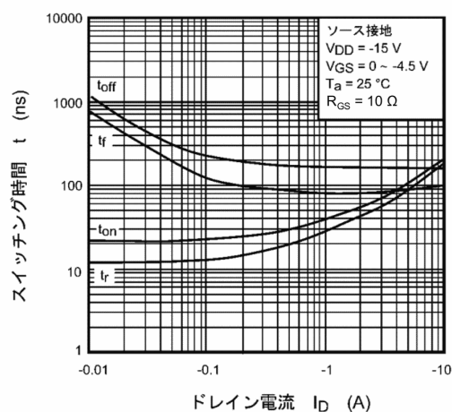
図 9.10 t - I_D
