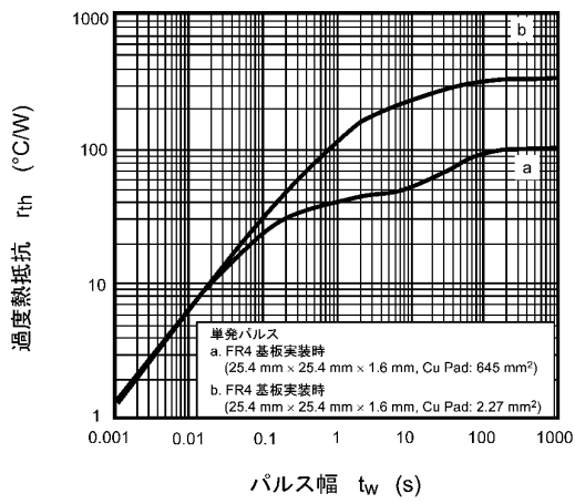
図 8.13 r_{th} - t_w
