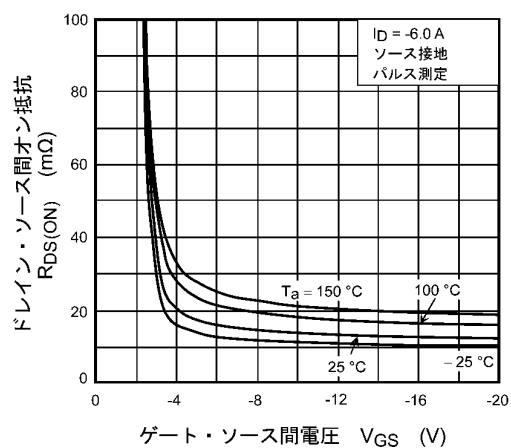
図 9.4 R_{DS(ON)} - V_{GS}
