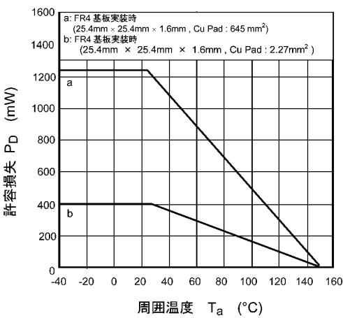
図 9.14 P_D - T_a
