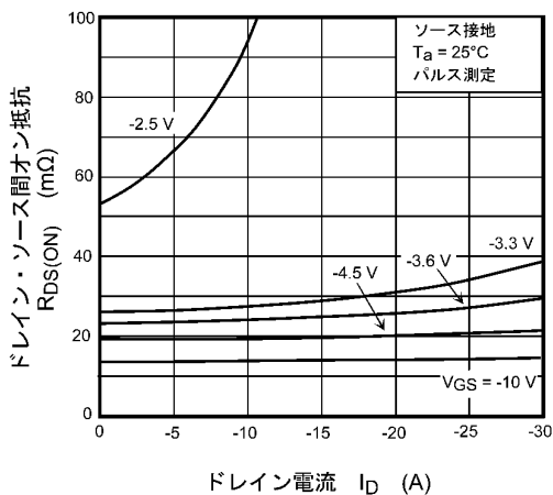
図 8.5 R_{DS(ON)} - I_D
