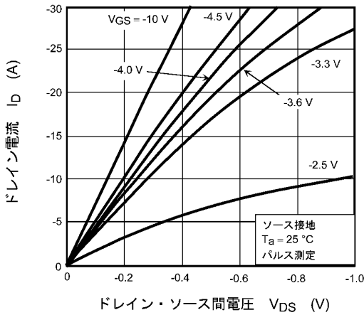
図 8.1 I_D - V_{DS}
