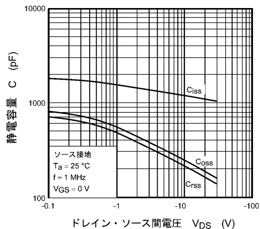
図 9.8 C - V_{DS}
