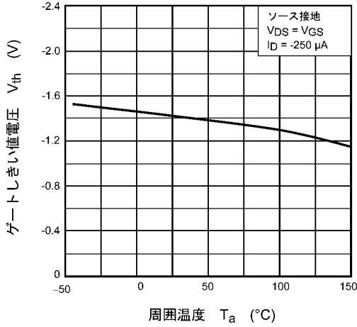
図 8.7 V_{th} - T_a
