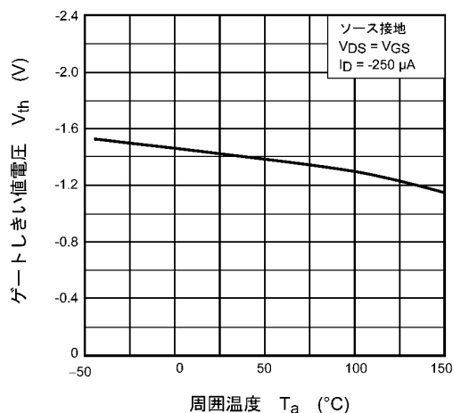
図 9.7 V_{th} - T_a
