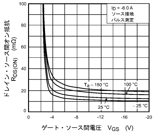
図 8.4 R_{DS(ON)} - V_{GS}
