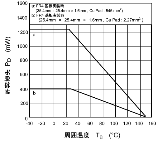
図 8.14 P_D - T_a
