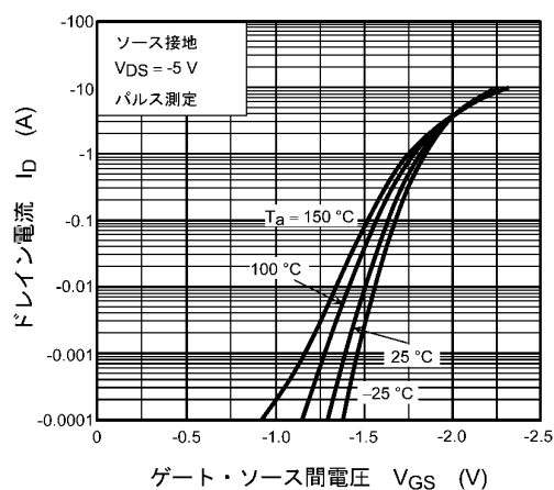
図 9.2 I_D - V_{GS}
