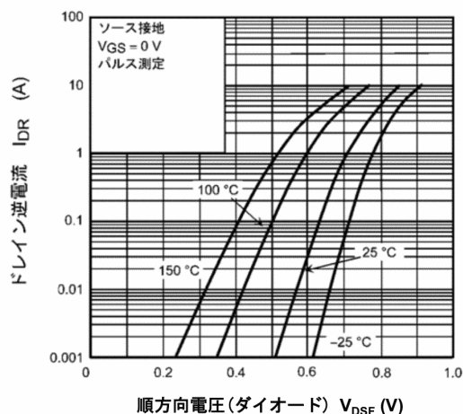
図 9.11 I_{DR} - V_{DSF}
