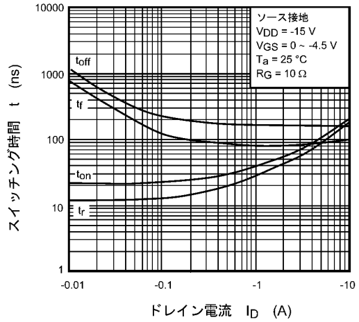
図 8.10 t - I_D
