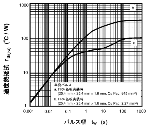
図 9.13 r_{th(j-a)} - t_w
