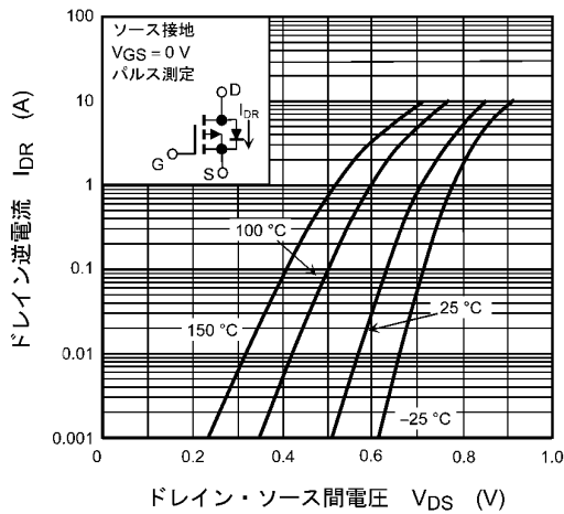
図 8.11 I_{DR} - V_{DS}
