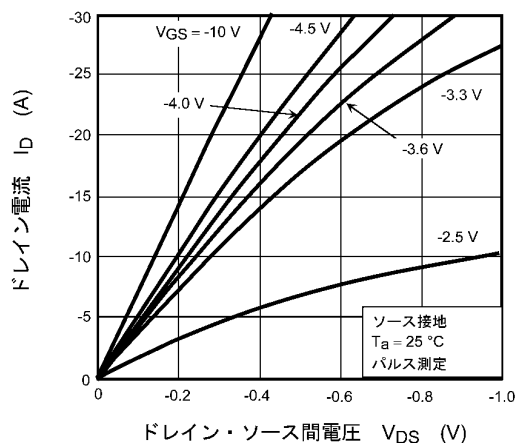
図 9.1 I_D - V_{DS}
