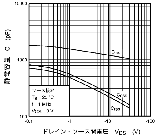
図 8.8 C - V_{DS}
