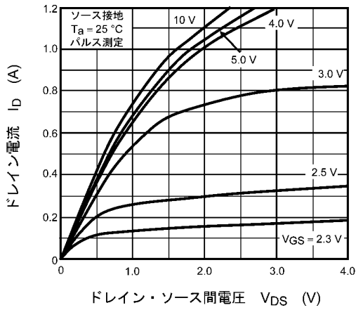
図 7.1 I_D - V_{DS}
