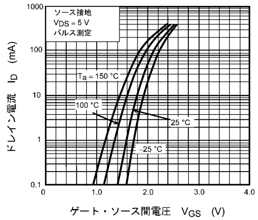
図 7.2 I_D - V_{GS}
