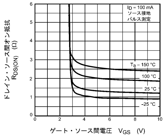
図 7.4 R_{DS(ON)} - V_{GS}
