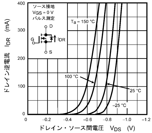
図 7.8 I_{DR} - V_{DS}
