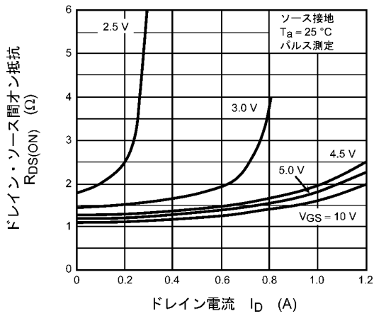
図 7.3 R_{DS(ON)} - I_D
