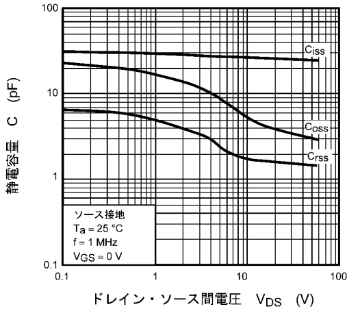
図 7.7 C - V_{DS}
