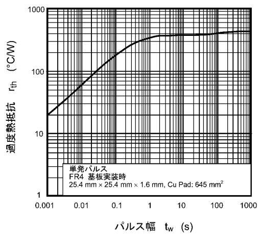
図 7.11 r_{th} - t_w
