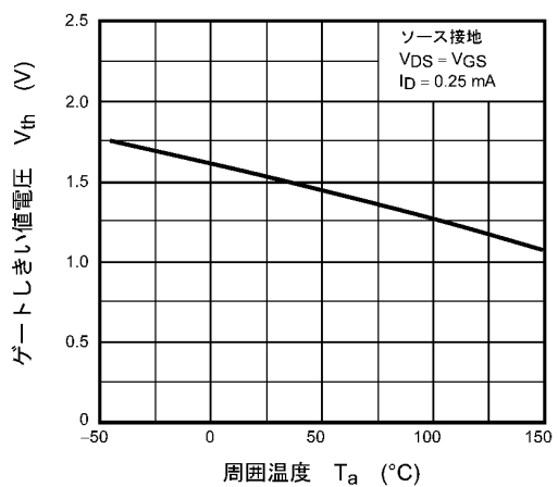
図 7.6 V_{th} - T_a
