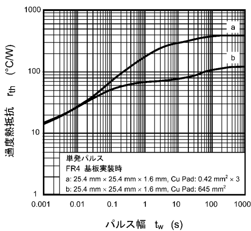
図 7.11 r_{th} - t_w
