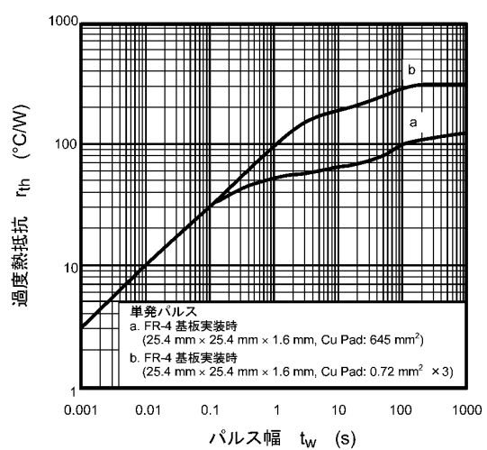
図 7.12 r_{th} - t_w
