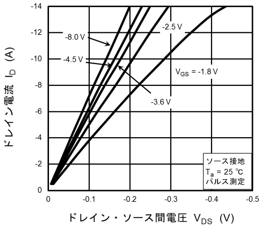
図 7.1 I_D - V_{DS}
