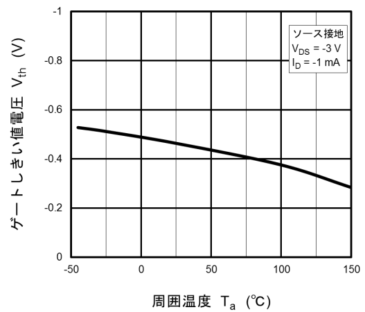
図 7.6 V_{th} - T_a
