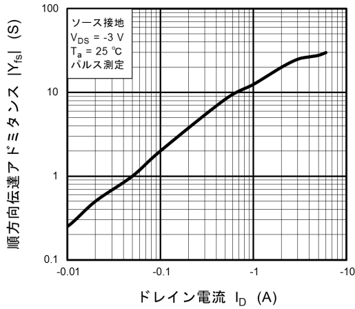
図 7.7 |Y_{fs}| - I_D
