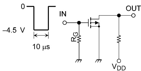
図 5.3.1 スwitchング時間の測定回路
