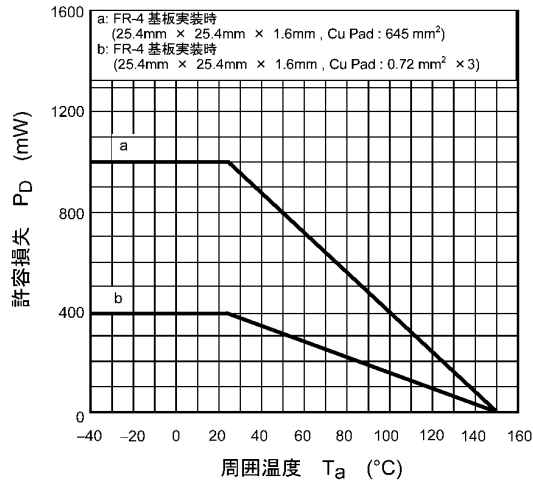
図 8.13 P_D - T_a
