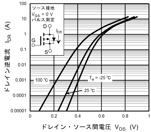
図 7.8 I_{DR} - V_{DS}
