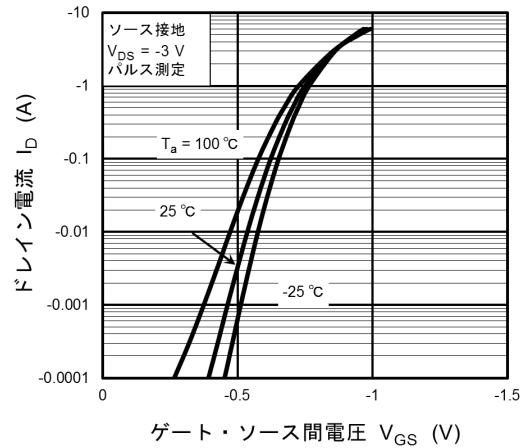
図 7.2 I_D - V_{GS}
