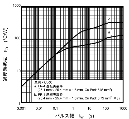
図 8.12 r_{th} - t_w
