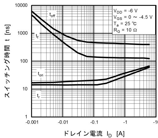
図 7.10 t - I_D
