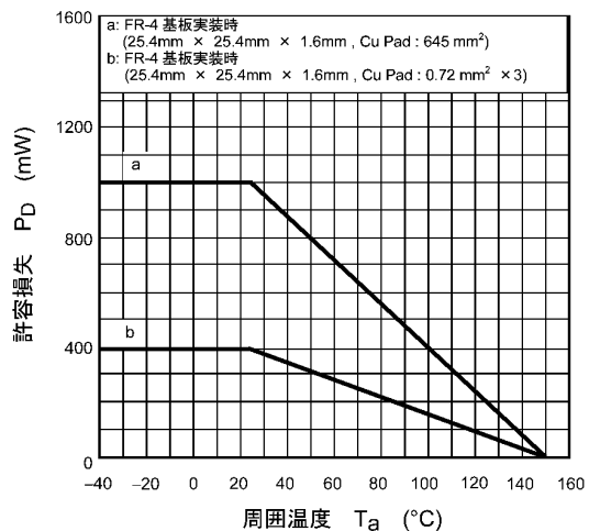
図 7.13 P_D - T_a
