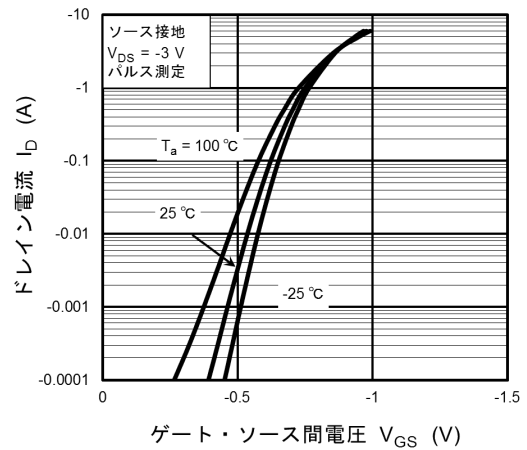
図 8.2 I_D - V_{GS}
