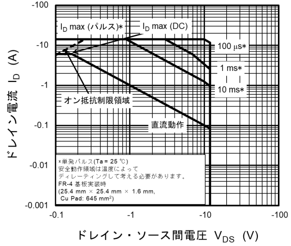
図 8.14 安全動作領域
