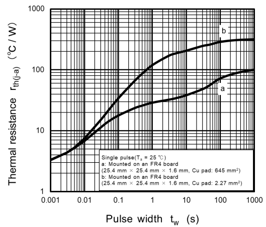
Fig. 9.12 r_{th(j-a)} - t_w
