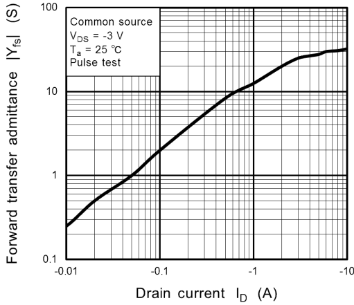
Fig. 9.7 |Y_{fs}| - I_D
