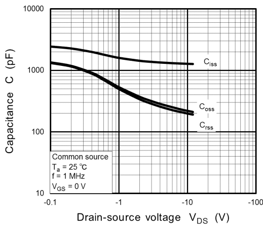
Fig. 9.9 C - V_{DS}
