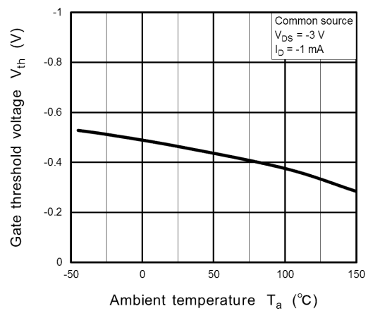
Fig. 9.6 V_{th} - T_a
