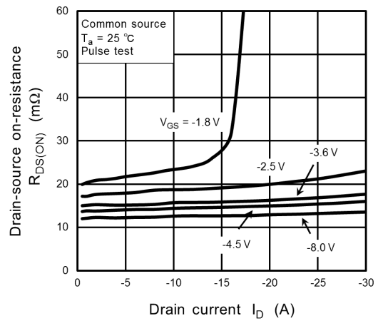
Fig. 9.4 R_{DS(ON)} - I_D
