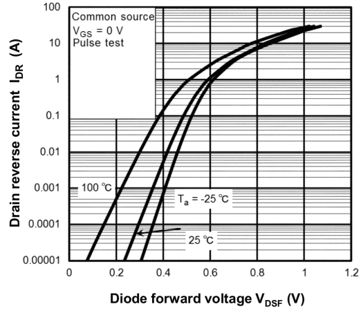
Fig. 9.8 I_{DR} - V_{DSF}
