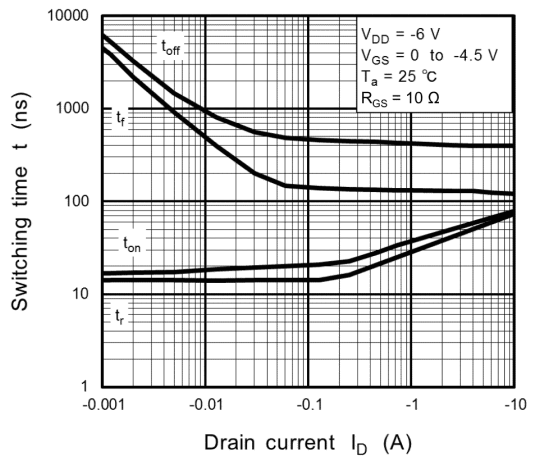
Fig. 9.10 t - I_D
