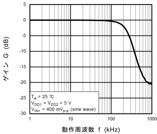
図 12.11 G[dB] - f
