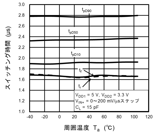
図 12.12 スイッチング時間 - T_a
