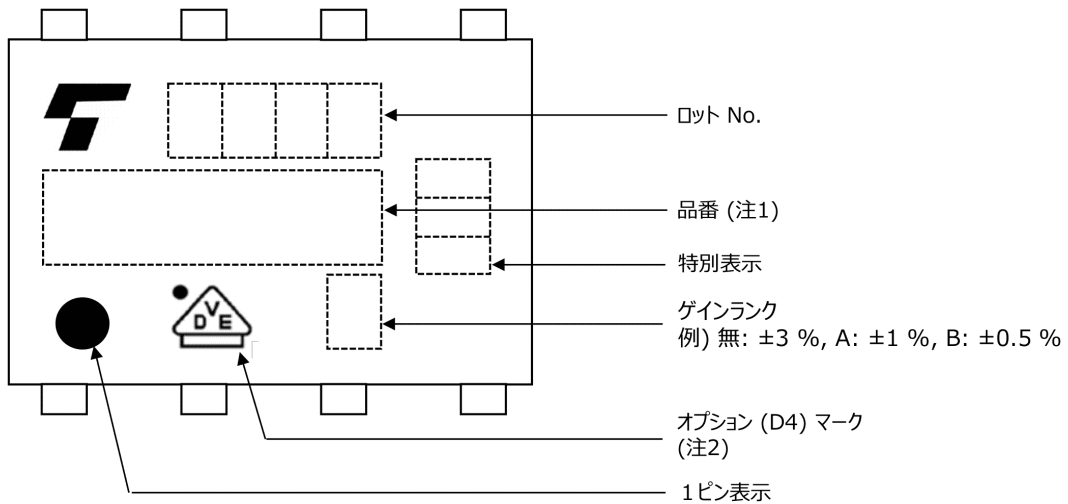
図 16.3 現品表示例
