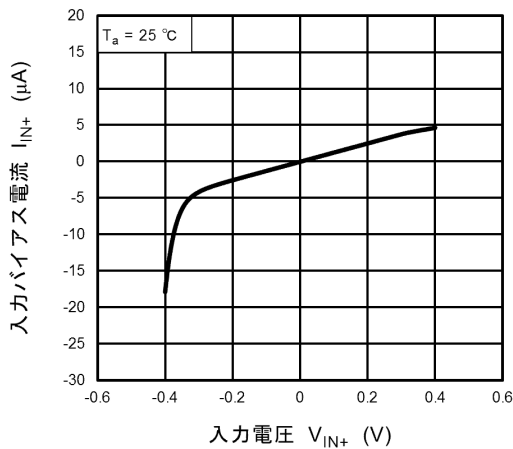
図 12.9 I_{IN+} - V_{IN+}
