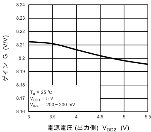
図 12.5 G - V_{DD2}
