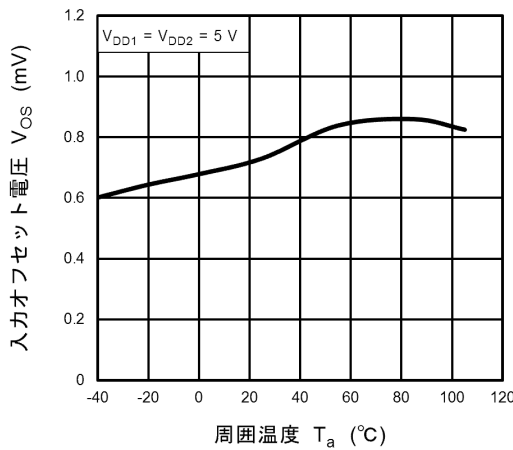
図 12.3 V_{OS} - T_a
