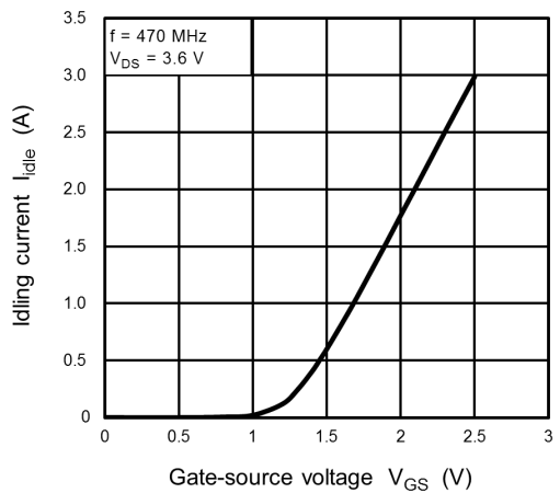
图 8.5 I_{idle} - V_{GS}
