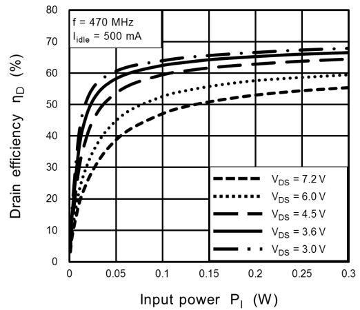
图 8.2 \eta_D - P_I
