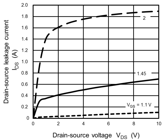
图 8.6 I_{DS} - V_{DS}
