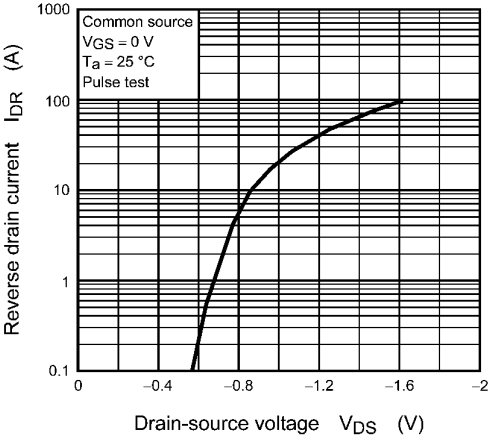
Fig. 8.8 I_{DR} - V_{DS}
