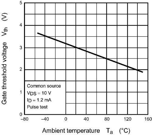
Fig. 8.11 V_{th} - T_a
