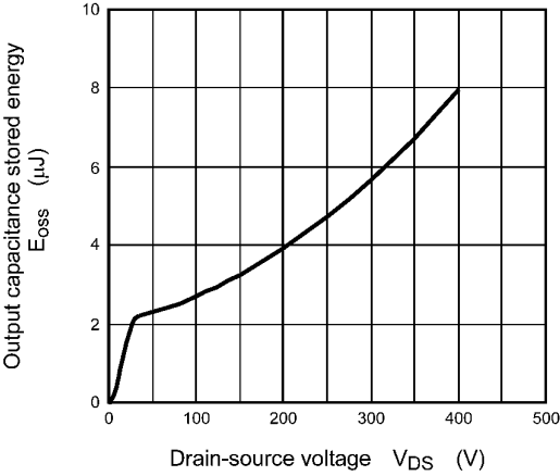
Fig. 8.10 E_{oss} - V_{DS}
