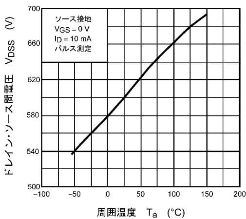
図 8.5 V_{DSS} - T_a
