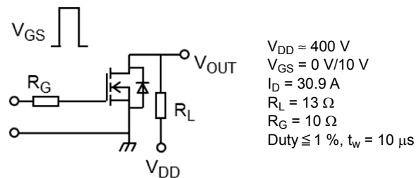
図 6.2.1 スwitchング時間の測定回路例
