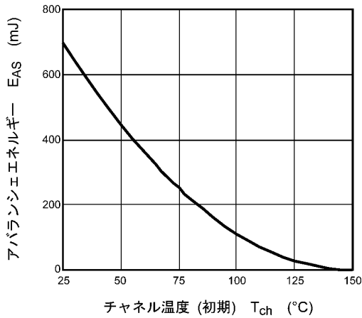
アバランシエエネルギー E_{AS} (mJ) チャンネル温度 (初期) T_{ch} (°C) 図 8.14 E_{AS} - T_{ch} (最大値 (保証値))
