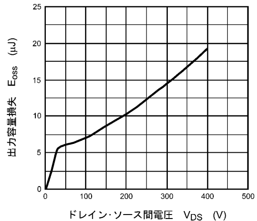
図 8.10 E_{oss} - V_{DS}
