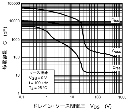
図 8.9 C - V_{DS}
