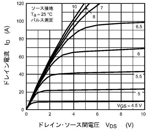
図 8.2 I_D - V_{DS}
