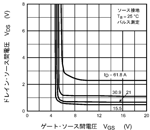
図 8.4 V_{DS} - V_{GS}
