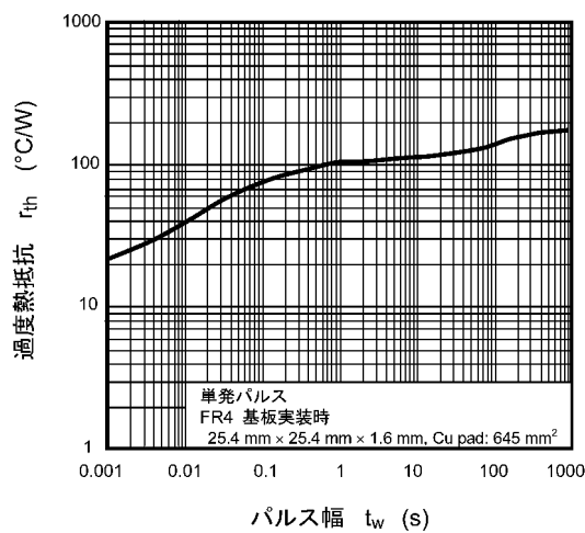
図 7.11 rth - tw
