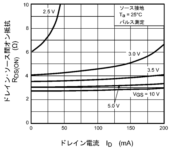
図 7.4 R_{DS(ON)} - I_D
