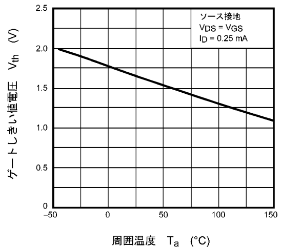
図 7.6 V_{th} - T_a
