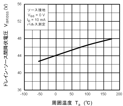
図 9.12 V_{(BR)DSS} - T_a
