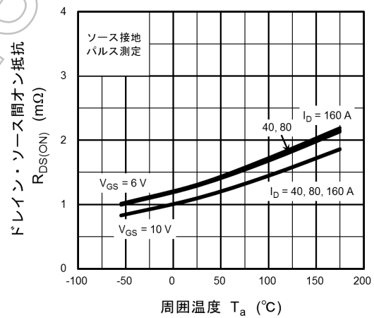
図 9.6 R_{DS(ON)} - T_a
