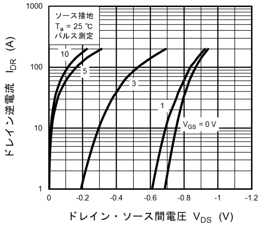
図 9.7 I_{DR} - V_{DS}
