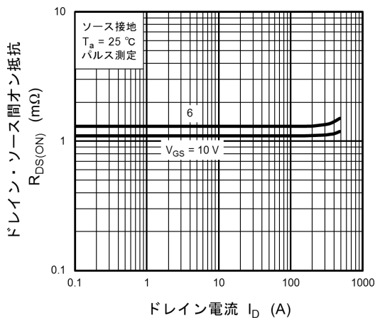
図 9.5 R_{DS(ON)} - I_D
