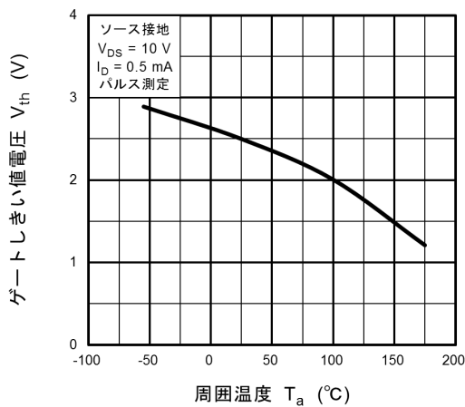
図 9.9 V_{th} - T_a
