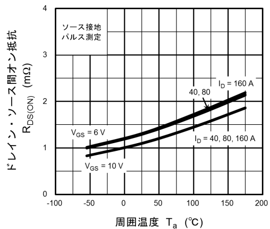
図 9.6 R_{DS(ON)} - T_a
