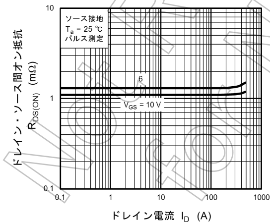
図 9.5 R_{DS(ON)} - I_D
