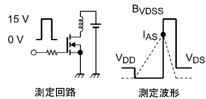
図 9.16 測定回路/測定波形
