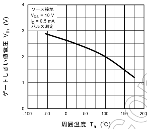
図 9.9 V_{th} - T_a
