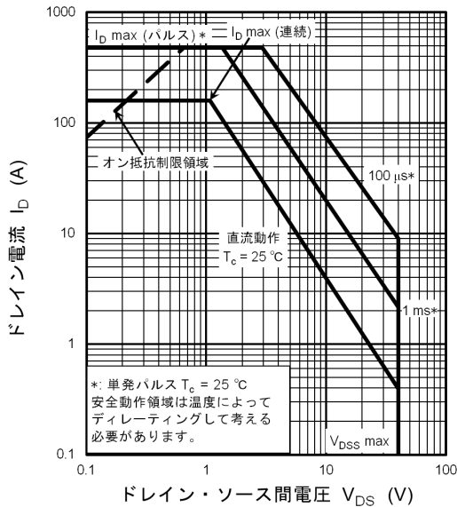
図 9.14 安全動作領域 (最大値 (保証値))
