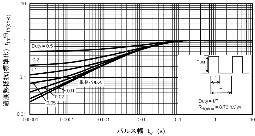
図 9.13 r_{th}/R_{th(ch-c)} - t_w (最大値 (保証値))
