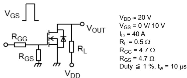
図 6.2.1 スwitching時間の測定回路例
