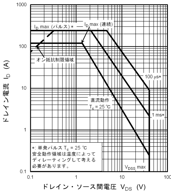
図 8.14 安全動作領域 (最大値 (保証値))
