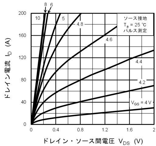
図 8.2 I_D - V_{DS}
