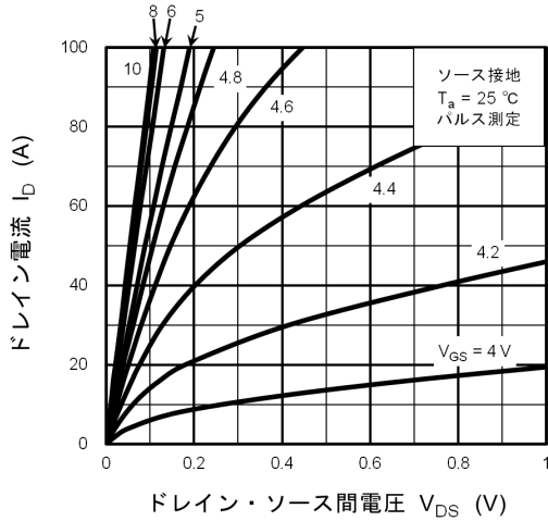
図 8.1 I_D - V_{DS}
