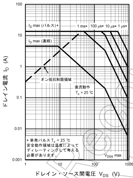
図 8.14 安全動作領域 (最大値 (保証値))
