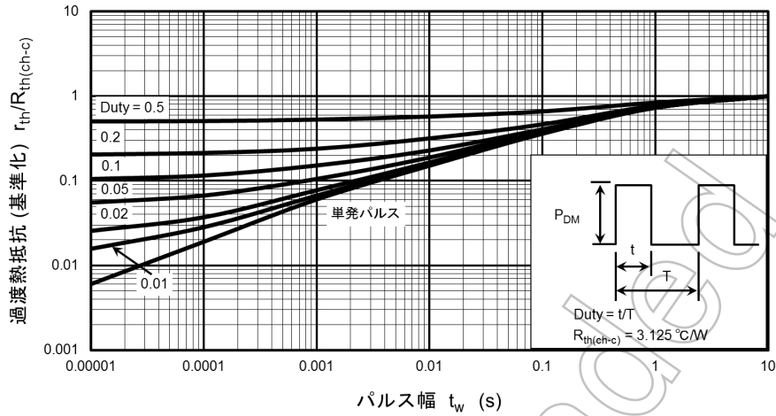
図 8.13 r_{tr}/R_{th(ch-c)} - t_w (最大値 (保証値))
