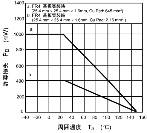
図 9.13 P_D - T_a
