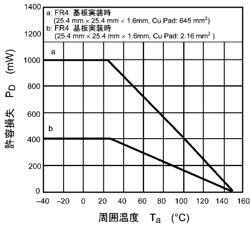
図 8.11 P_D - T_a
