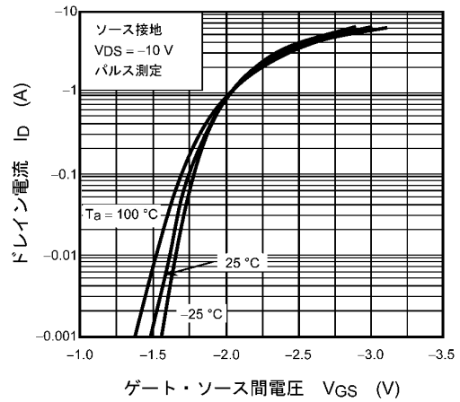
図 8.2 I_D - V_{GS}
