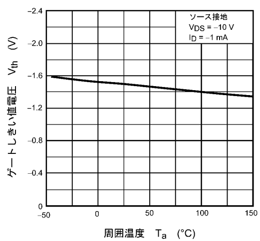
図 8.6 V_{th} - T_a
