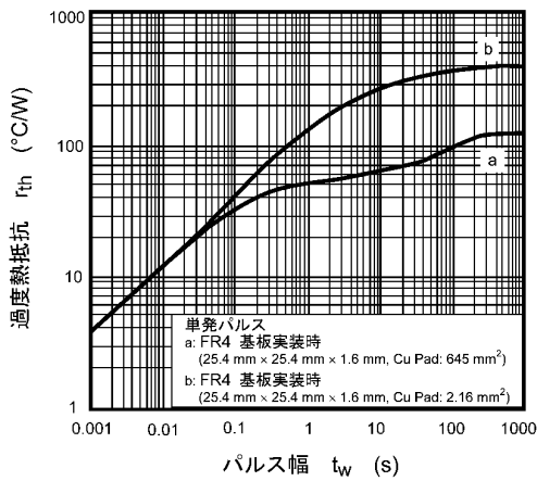
図 9.11 r_{th} - t_w
