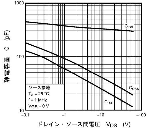
図 9.8 C - V_{DS}
