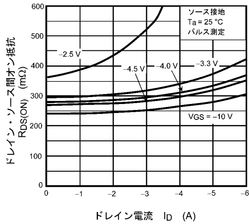
図 8.4 R_{DS(ON)} - I_D
