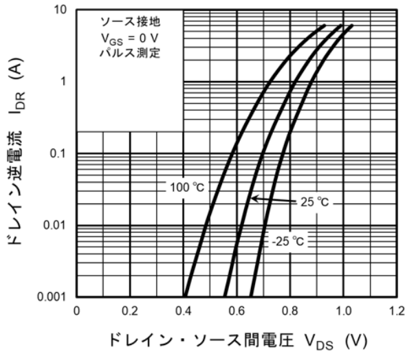
図 8.7 I_{DR} - V_{DS}
