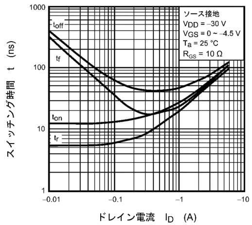
図 9.10 t - I_D
