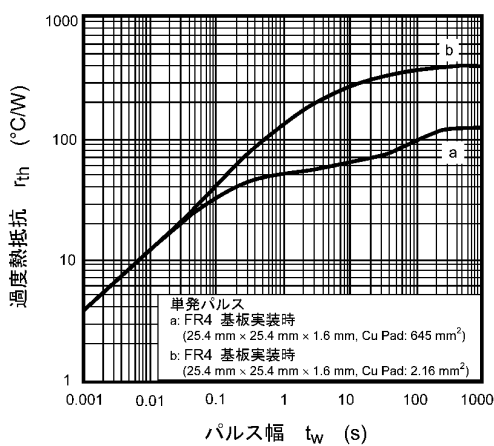
図 8.11 r_{th} - t_w
