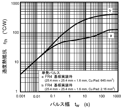
図 7.11 r_{th} - t_w
