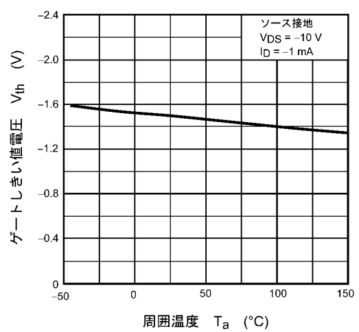
図 8.6 V_{th} - T_a
