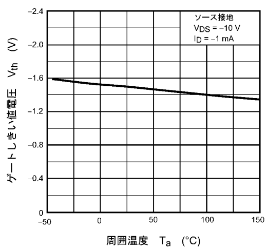
図 7.6 V_{th} - T_a
