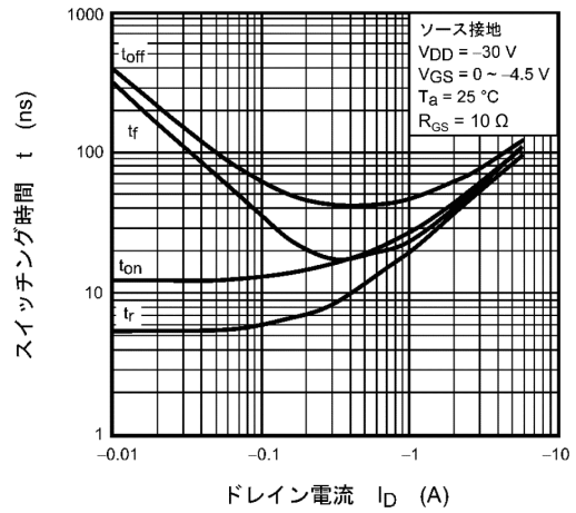
図 8.10 t - I_D
