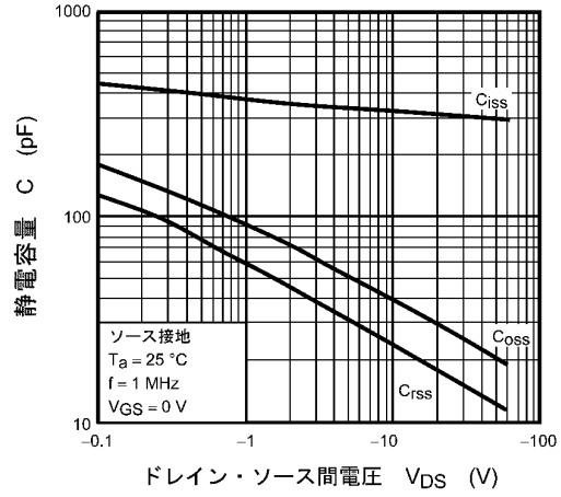
図 7.8 C - V_{DS}
