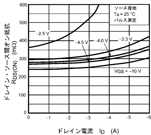
図 7.4 R_{DS(ON)} - I_D
