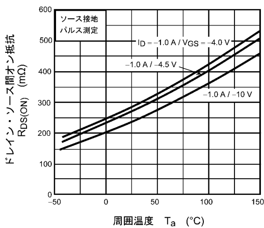
図 8.5 R_{DS(ON)} - T_a
