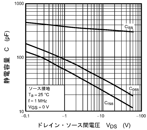
図 8.8 C - V_{DS}
