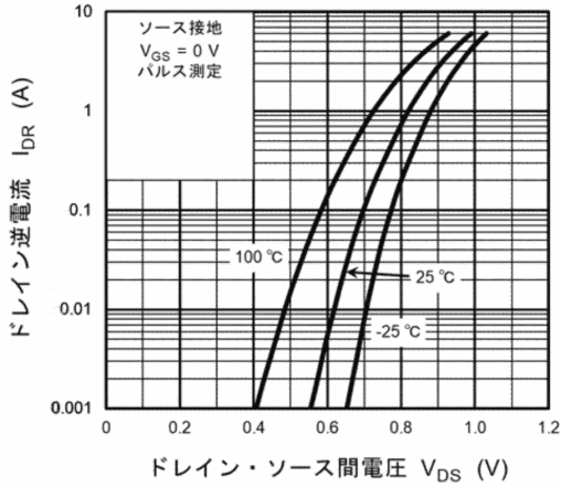
図 9.7 I_{DR} - V_{DS}
