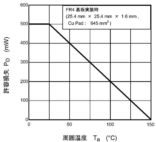
図 7.12 P_D - T_a
