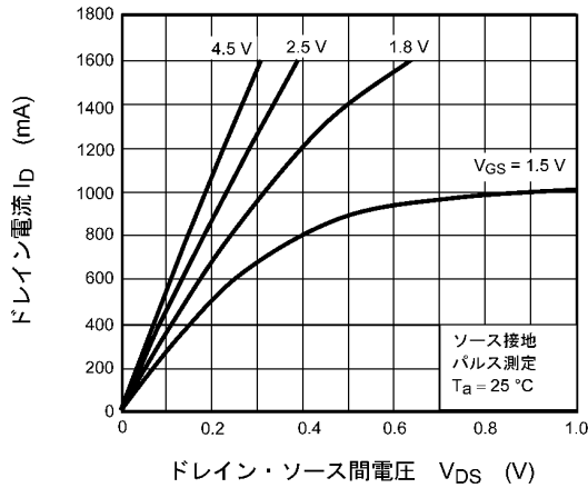
図 7.1 I_D - V_{DS}
