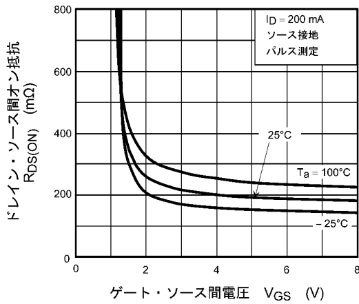
図 7.3 R_{DS(ON)} - V_{GS}
