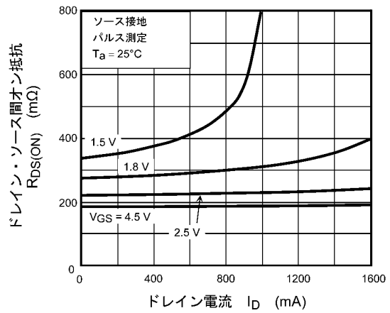
図 7.4 R_{DS(ON)} - I_D
