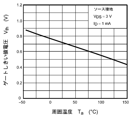
図 7.6 V_{th} - T_a
