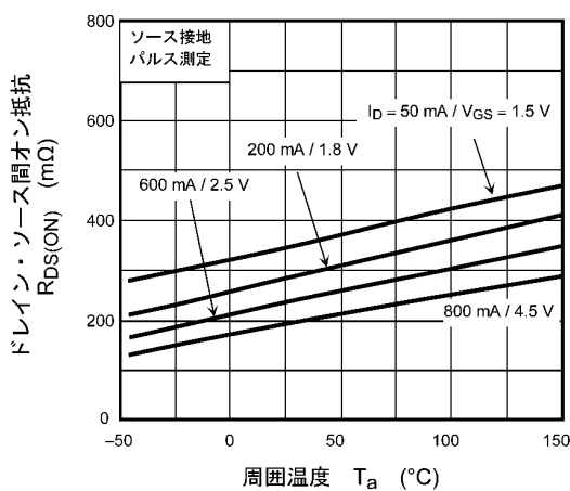
図 7.5 R_{DS(ON)} - T_a
