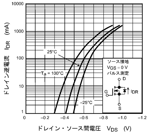
図 7.8 I_{DR} - V_{DS}
