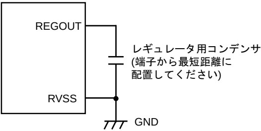
図 1-3 レギュレータ用コンデンサ接続
