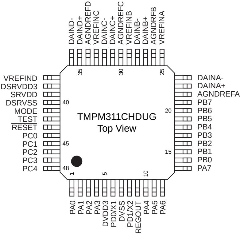
図 1-2 ピン配置図
