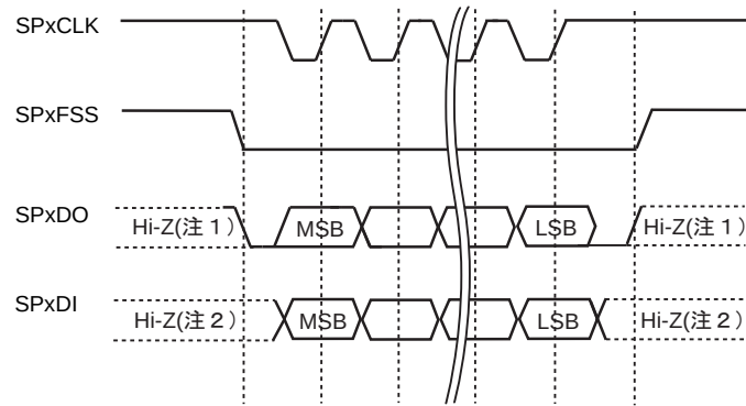
図 14-9 SPI フレームフォーマット (<SPO>=1 & <SPH>=1)
