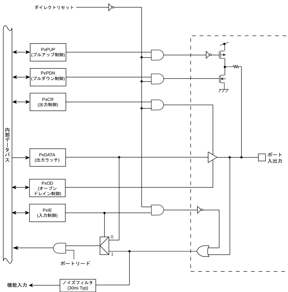
図 10-3 タイプ FT4
