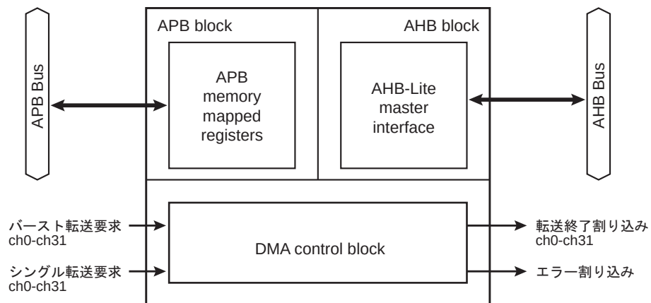
図 9-1 μDMA ブロック図(ユニット共通)
