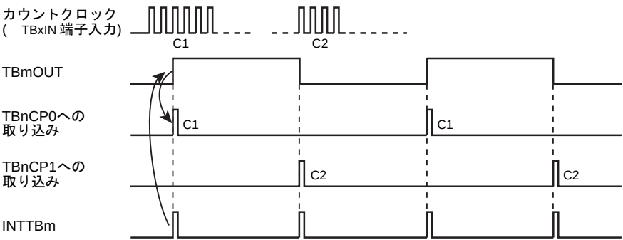
図 11-6 周波数測定
