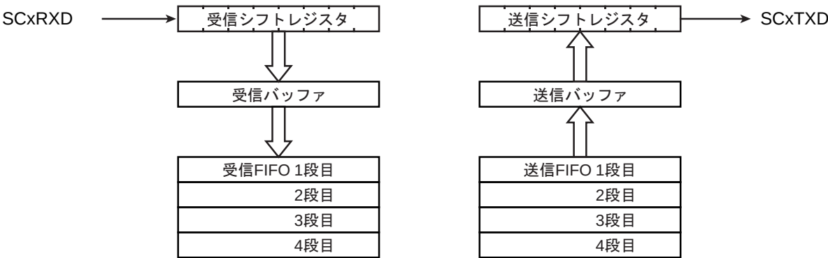
図 13-4 バッファと FIFO の構成
