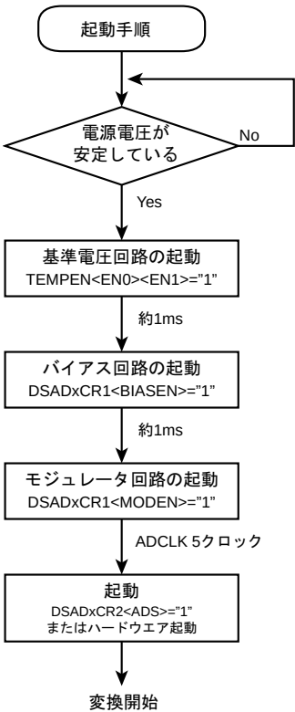
図 15-2 起動手順
