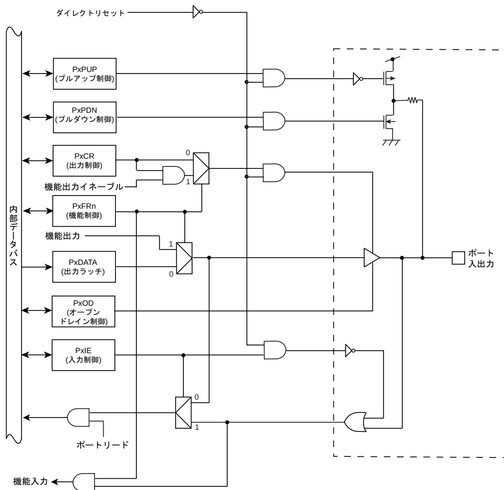
図 10-2 タイプ FT2
