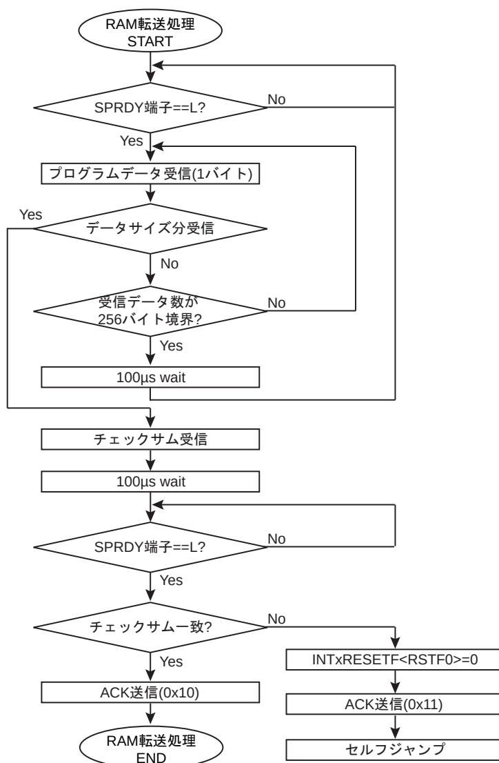
図 6-4 RAM 転送データの受信フローチャート
