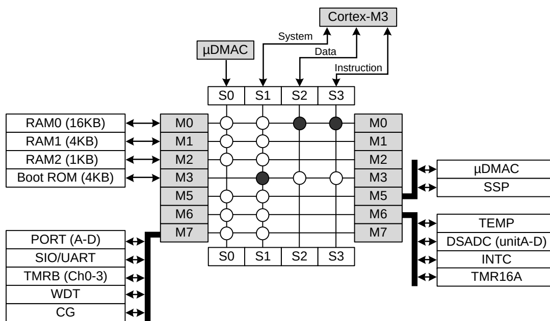
図 4-1 バス構成
