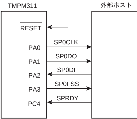
図 6-1 ブートプログラムの使用端子
