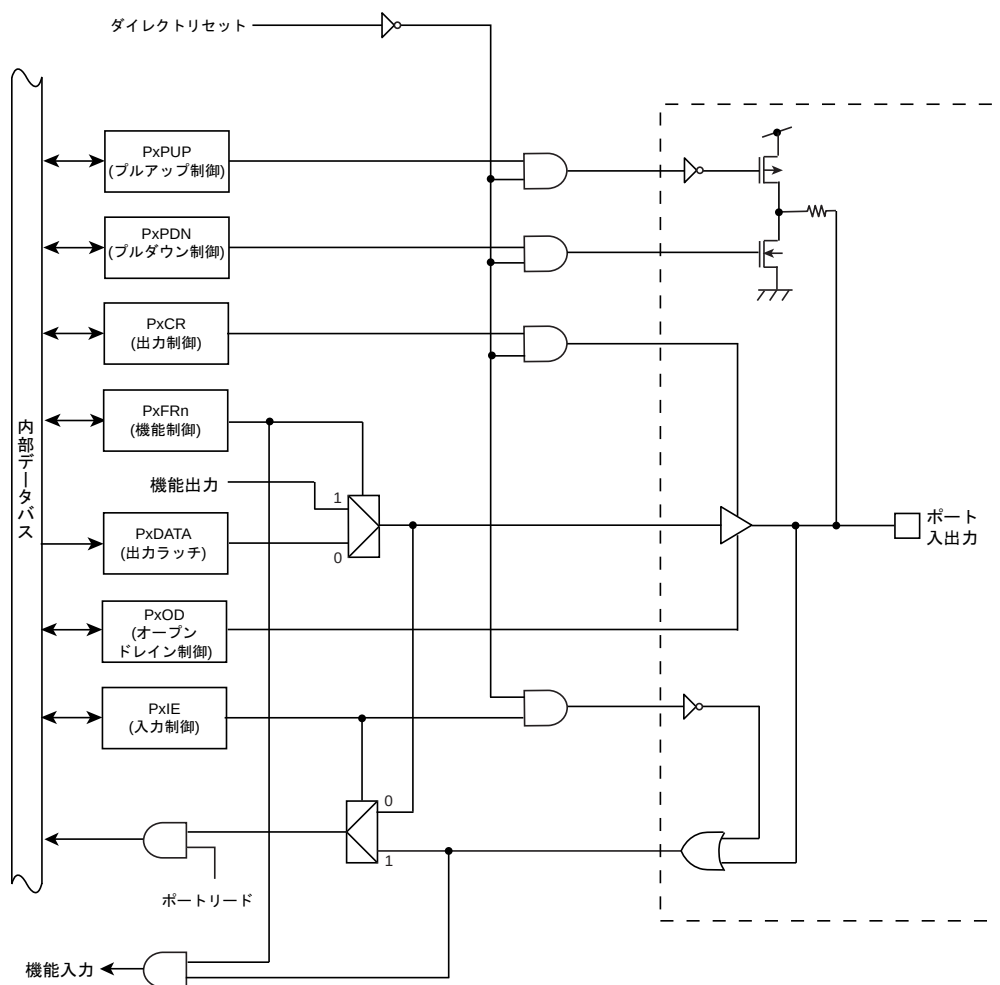
図 10-1 タイプ FT1
