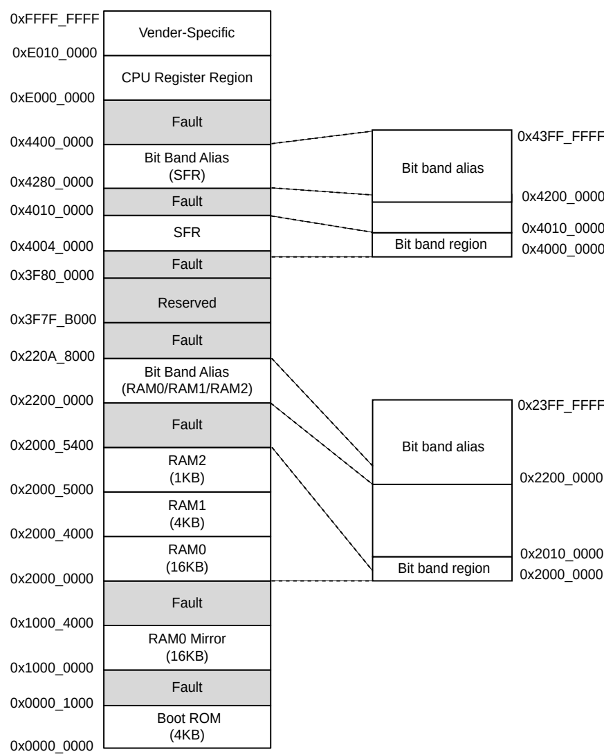
図 4-2 メモリマップ
