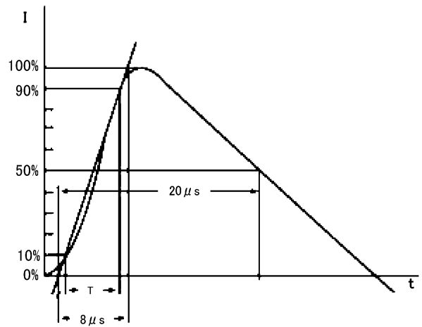
図 9.2 IEC61000-4-5準拠 8/20 \mu\text{s} (Ed.2)
