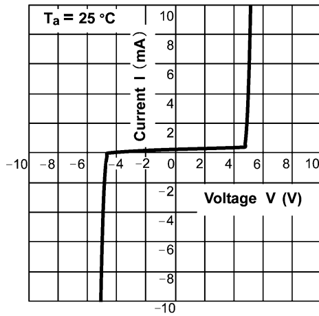
図 7.1 I - V
