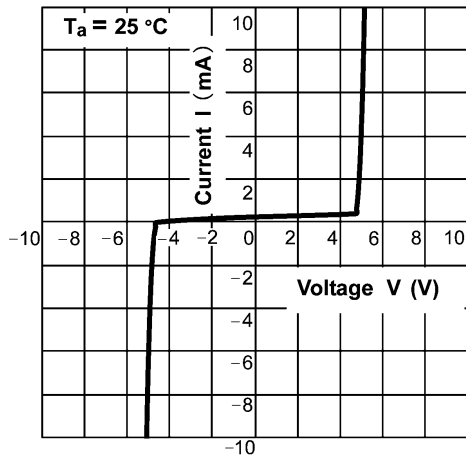
図 8.1 I - V
