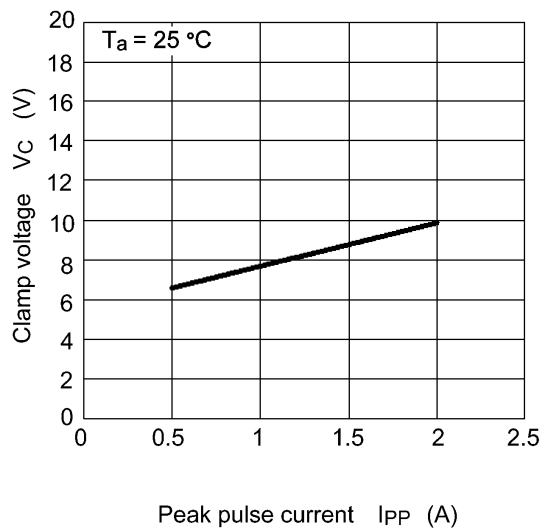
図 9.1 V_C - I_{PP}
