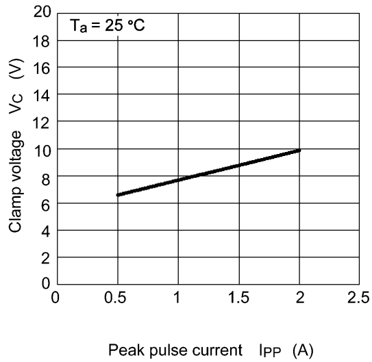
図 8.1 V_C - I_{PP}
