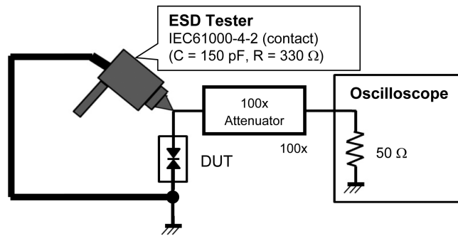
図 11.5 IEC61000-4-2準拠 (接触放電)
