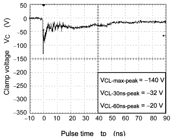
図 11.4 -15 kV
