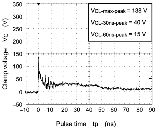
図 11.3 +15 kV
