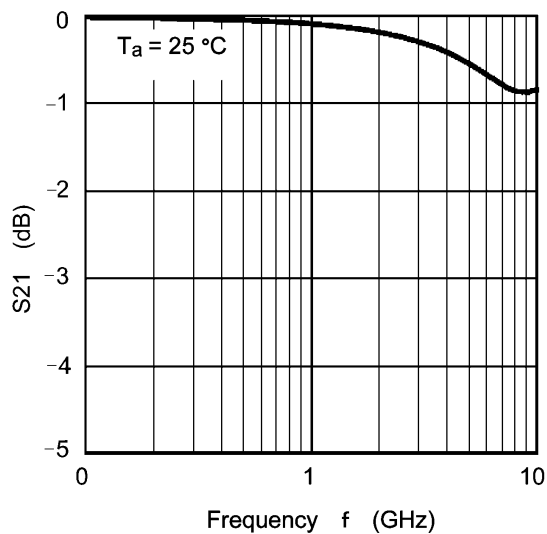
図 10.1 S21 - f
