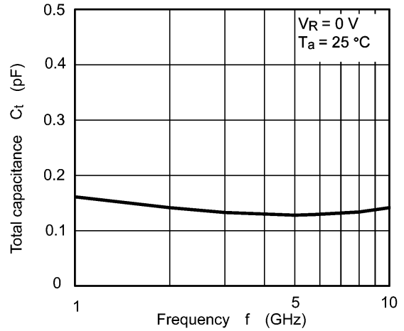
図 8.4 C_t - f
