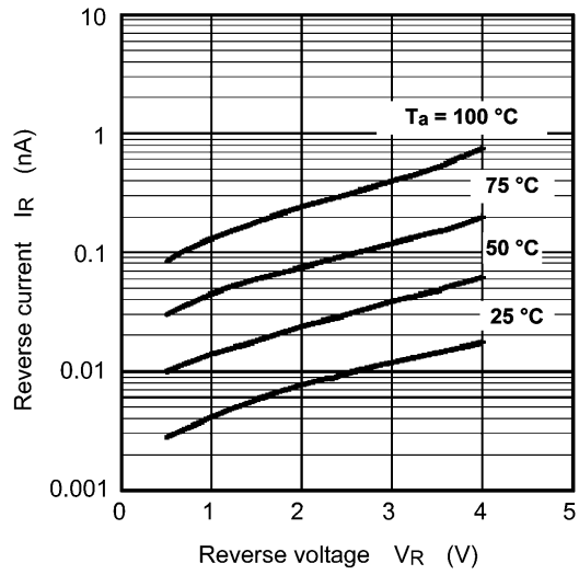
図 8.2 I_R - V_R
