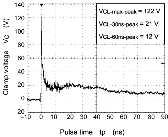
図 11.1 +8 kV
