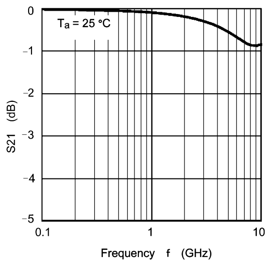
図 9.1 S21 - f
