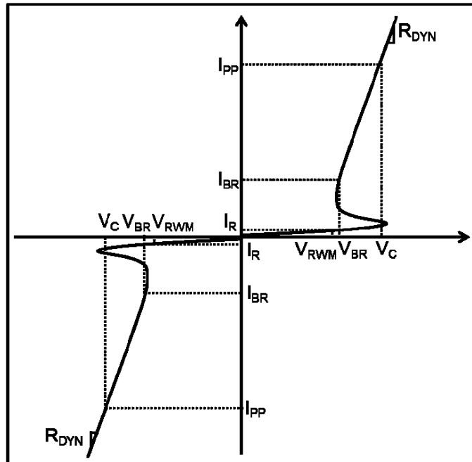
図 4.1 電気的特性の定義
