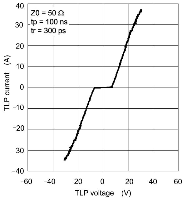
図 9.3 TLP
