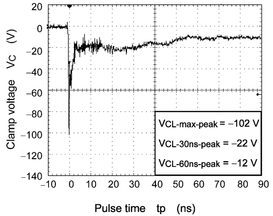
図 11.2 -8 kV
