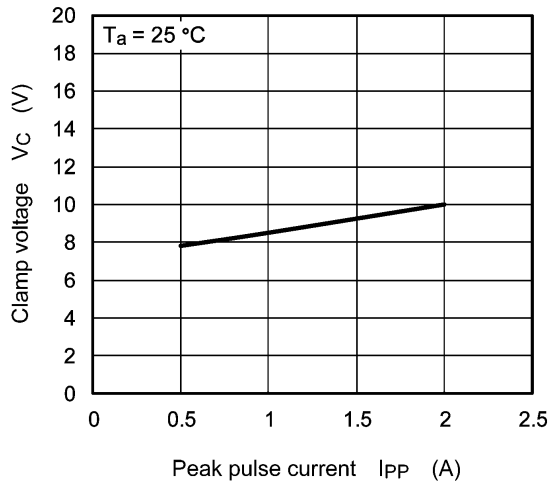
Fig. 8.1 V_C - I_{PP}
