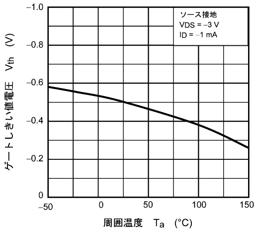
図 8.7 V_{th} - T_a
