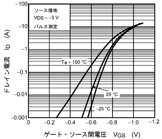
図 8.2 I_D - V_{GS}
