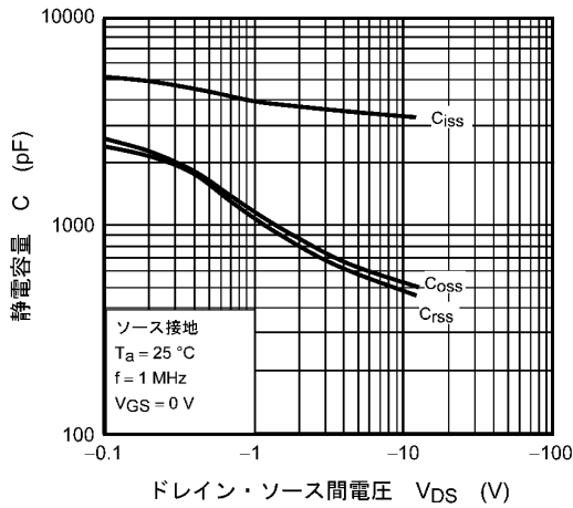
図 8.9 C - V_{DS}
