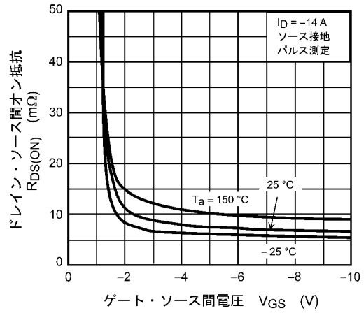
図 8.4 R_{DS(ON)} - V_{GS}
