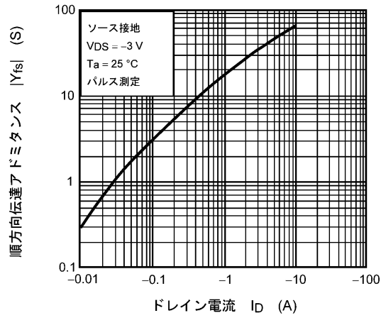
図 8.8 |Y_{fs}| - I_D
