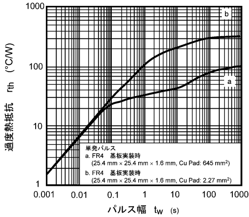
図 8.13 r_{th} - t_w
